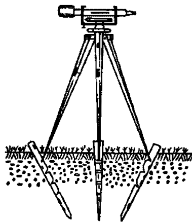
Рисунок 9. Установка нивелира на крутых косогорах и на заболоченной почве.
