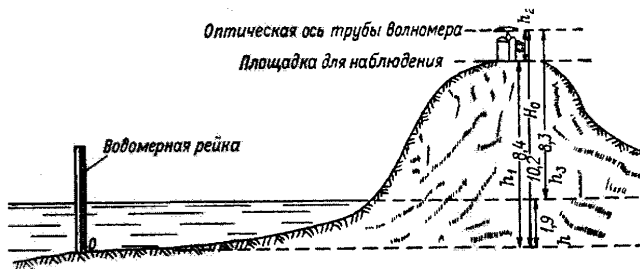
Рисунок 15 – Схема нивелирования водомерного пункта.
