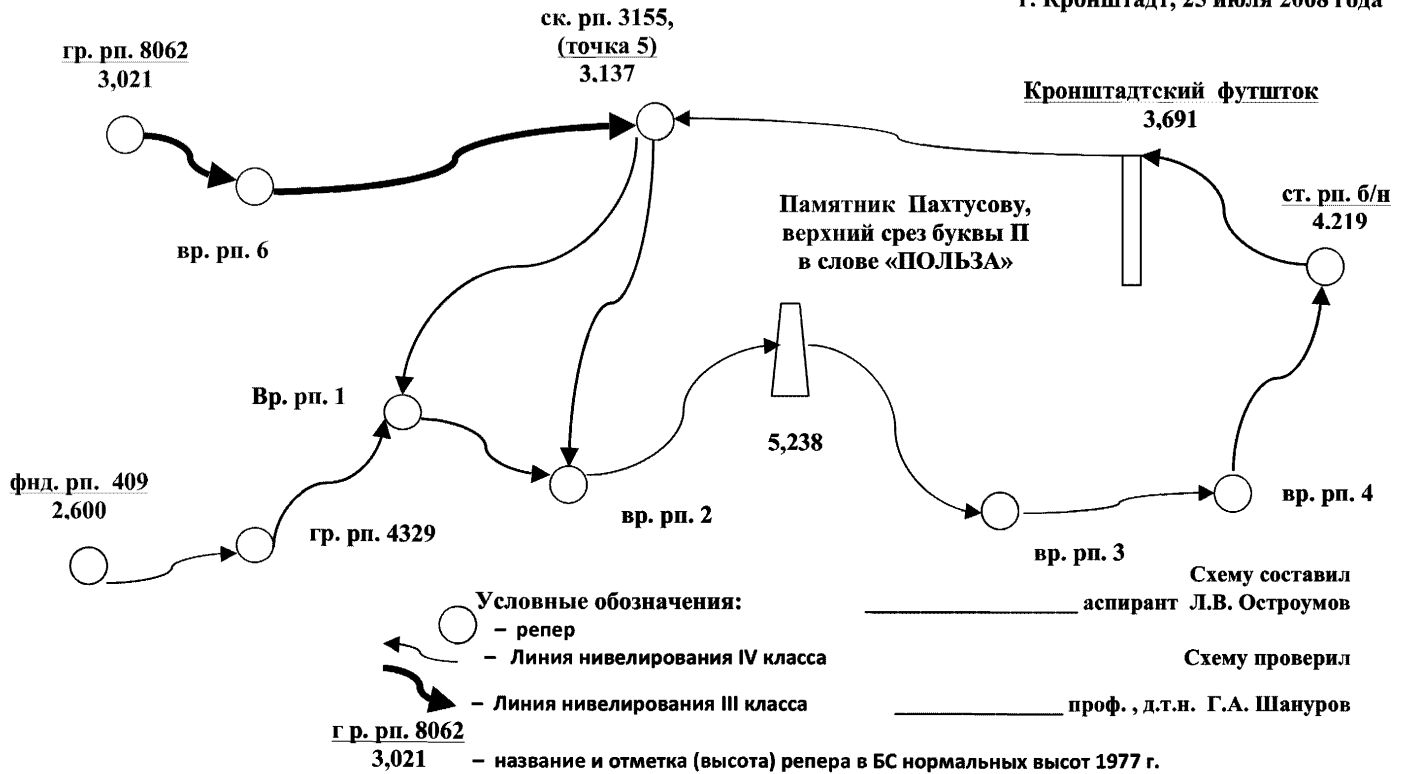
Рисунок В.1 – Схема нивелирного хода
