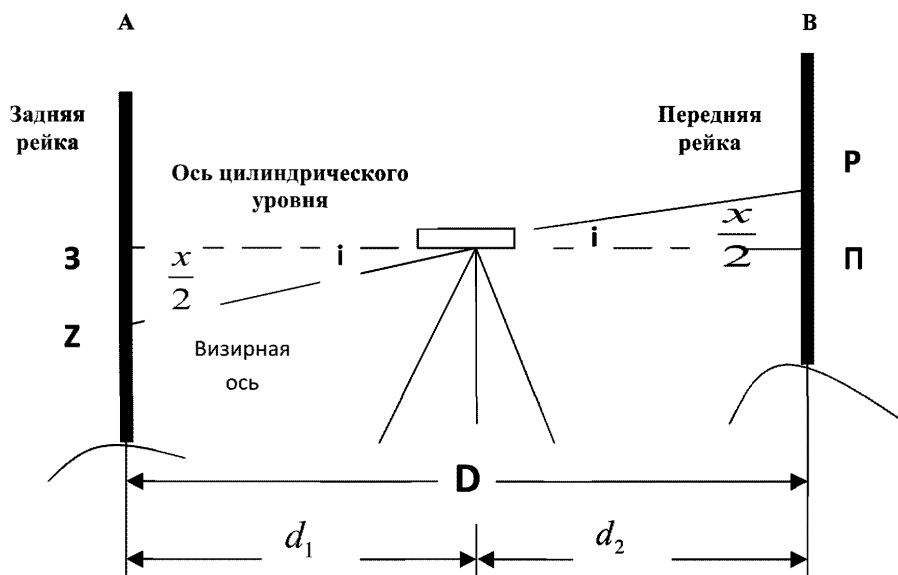
Рисунок А.1 – Определение превышения при нивелировании из середины
