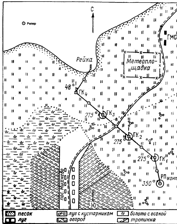
Рисунок 16 – Схема нивелирного хода от рабочего (контрольного) репера.
