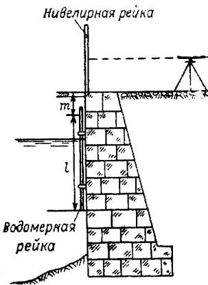
Рисунок 13 – Нивелирование водомерной рейки на устой моста.
