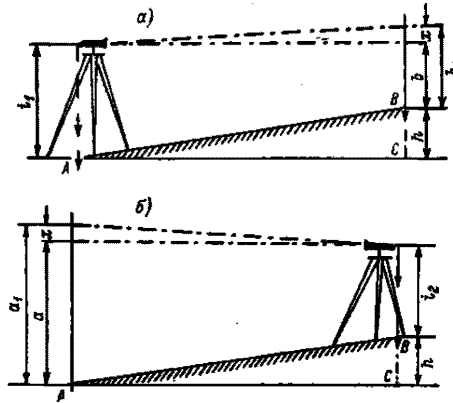
Рисунок 6 – Проверка нивелира.
