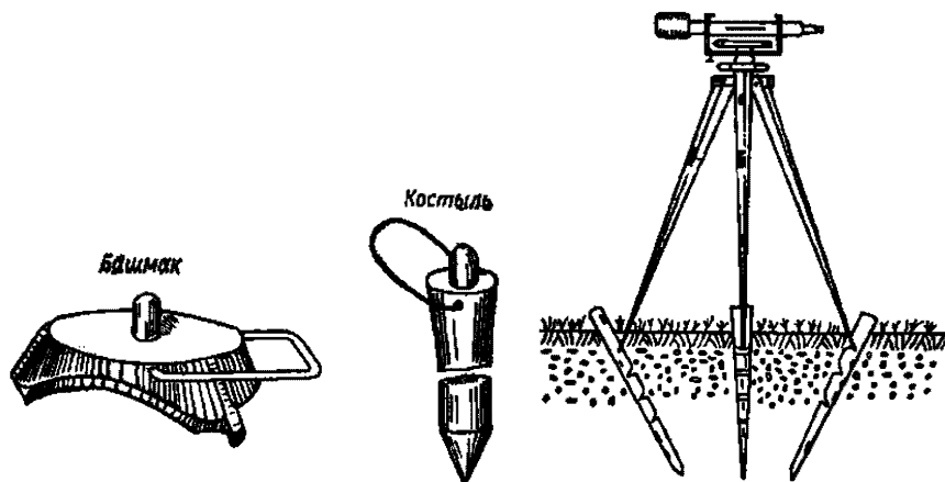
Рисунок 8. Приспособления для установки нивелирной рейки.
