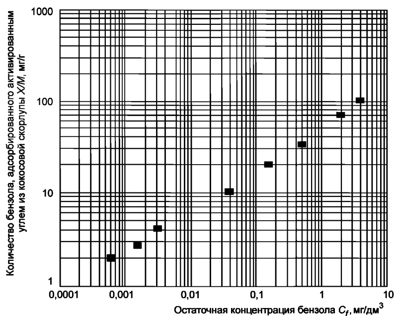
Рисунок 1 — Изотерма адсорбции
