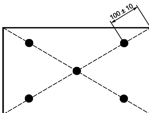
Рисунок В.1 — Расположение точек на поверхности стекла для измерения напряжения
