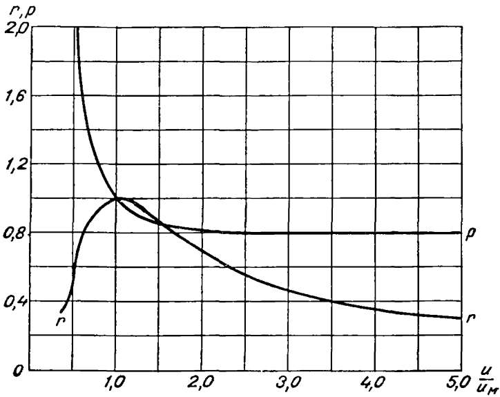
Рис. 4. График для определения вспомогательных величин r и \rho , используемых при расчете концентраций при неблагоприятных метеорологических условиях и скорости ветра u , отличающейся от u_M .
