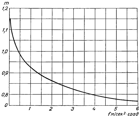
Рис. 2. График для определения коэффициента m , учитывающего условия выхода газозвдушной смеси из устья источника.
