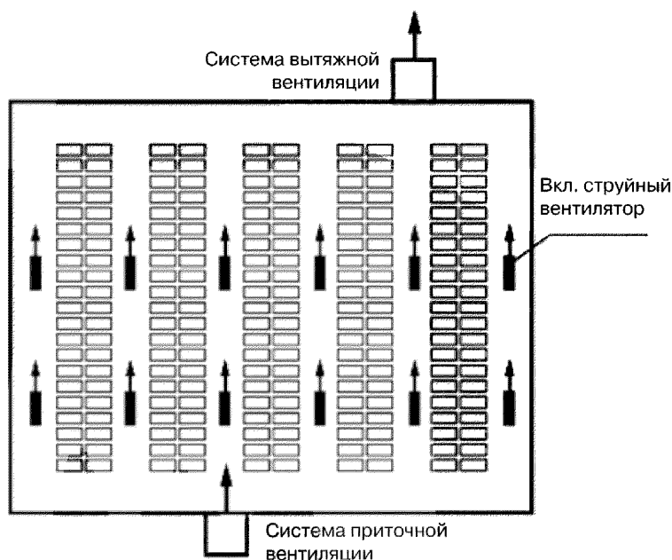
Рисунок 5.2 – Вентиляционная система автостоянки в штатном режиме
