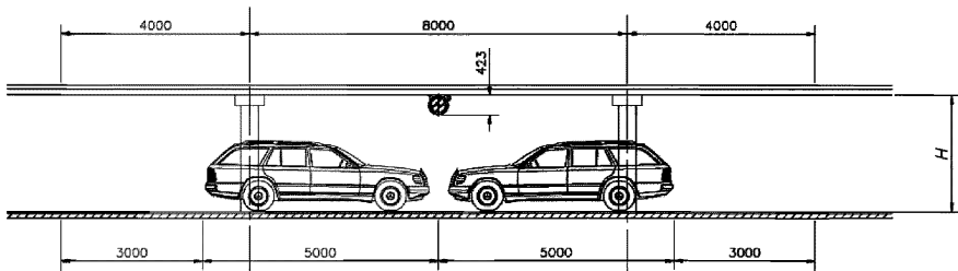
Рисунок 5.8 – Расположение струйных вентиляторов над парковочными местами
