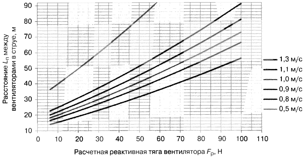
Рисунок 6.9 – График зависимости продольного расстояния между вентиляторами L_{п} (в струе) от расчетной реактивной тяги F_p вентилятора при различных значениях v_{x \min}
