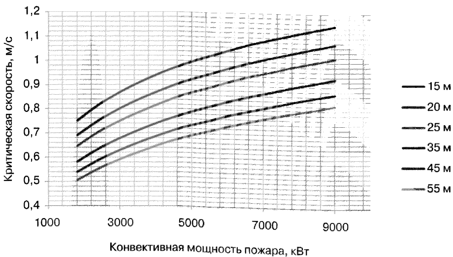
Рисунок 6.3 – График зависимости критической скорости от конвективной мощности пожара при различных габаритных размерах B автостоянки, при Fr = 6,0
