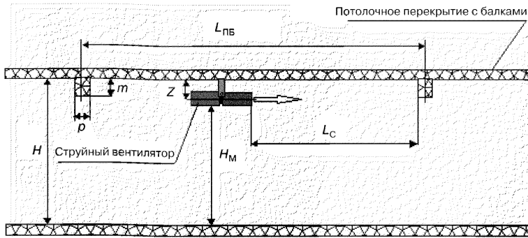
Рисунок 5.4 – Схема расположения струйного вентилятора под потолочным перекрытием
