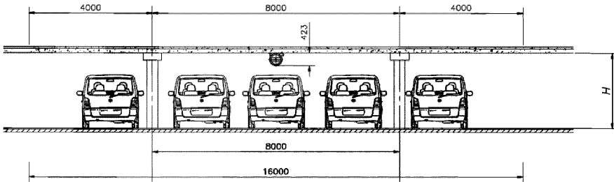
Рисунок 5.7 – Расположение струйных вентиляторов над парковочными местами
