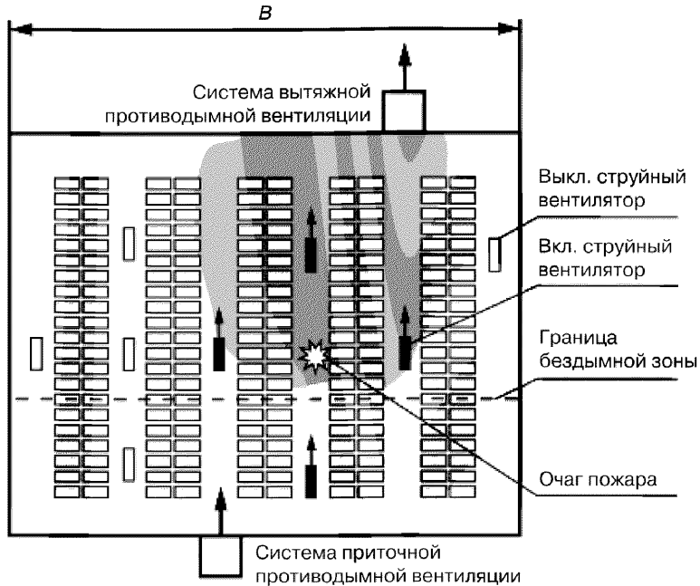
Рисунок 5.1 – Вентиляционная система автостоянки в режиме дымоудаления при продольной схеме противодымной вентиляции
