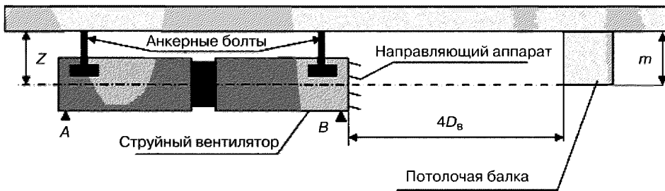
Рисунок 7.1 – Схема монтажа струйного вентилятора
