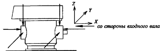
Рис. 9.9.2 Точки измерения вибрации винторулевых колонок
