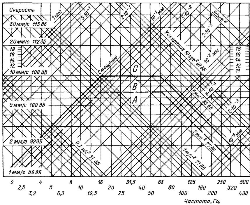
Рис. 9.5.1 Нормы вибрации насосов мощностью 15 — 75 кВт:
