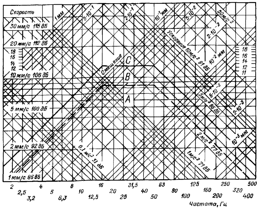
Рис. 9.5.3 Нормы вибрации вентиляторов:
