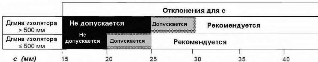
Рисунок 11 — Рекомендации по выбору межреберного расстояния
