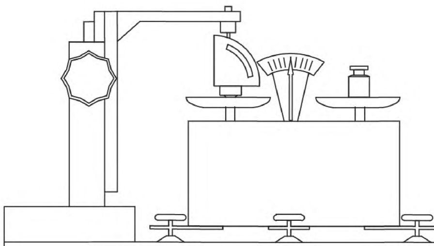
Рисунок 3 — Аппаратура для калибровки пружины дюрометра
