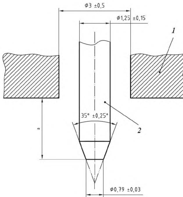
Рисунок 1 — Индентор для дюрометра типа А
