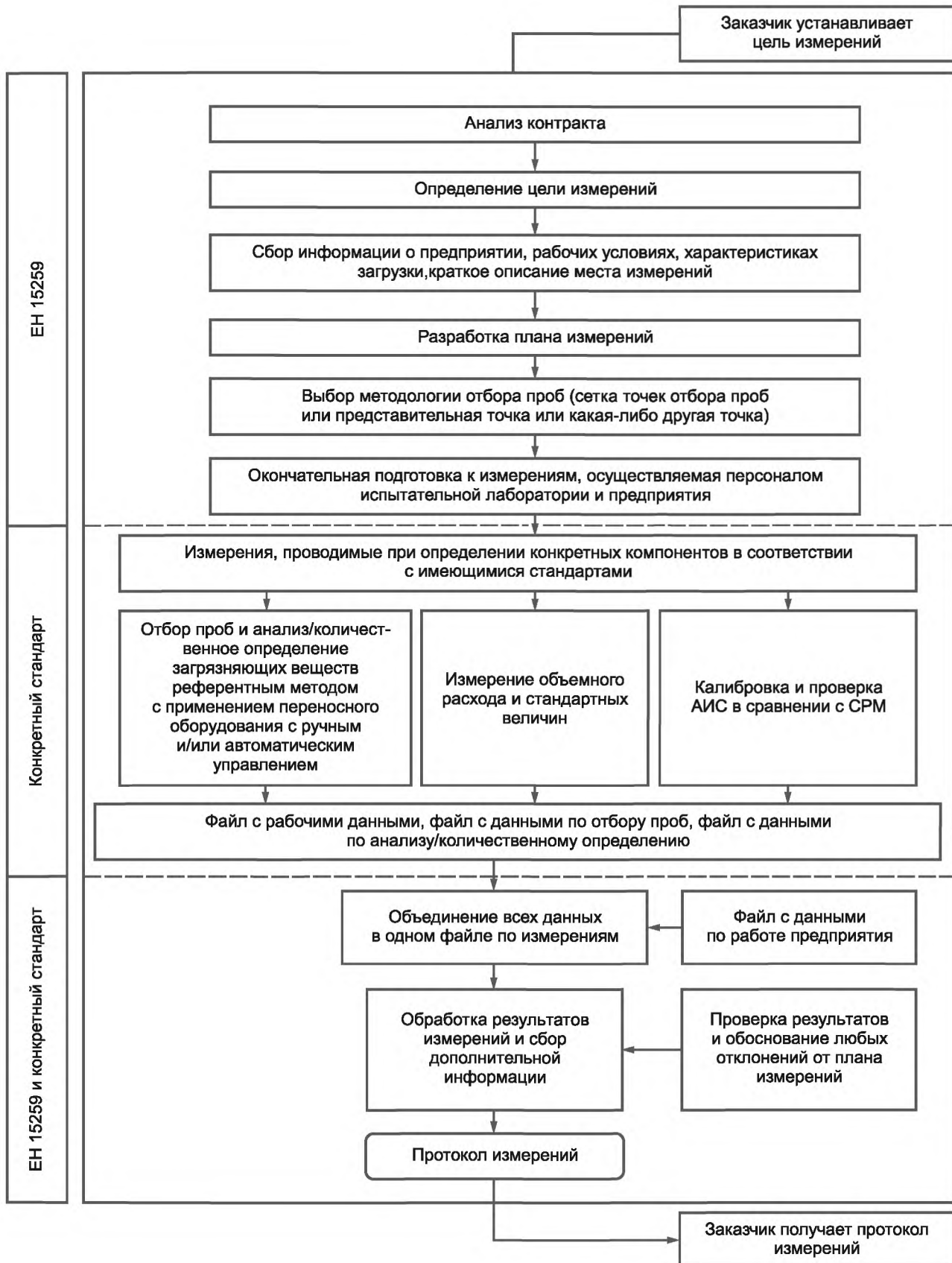
Рисунок 1 — Основные этапы периодических измерений выбросов стационарных источников
