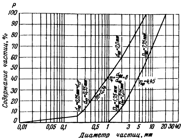
Рис. 31. Гранулометрический состав грунта основания и щебенистого грунта, предназначенного для фильтра из пористого бетона.
