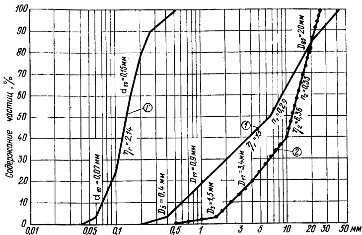
Рис. 25. Гранулометрический состав грунтов \Gamma — грунт тела плотины; 1, 2 — карьерные грунты для фильтровой подготовки
