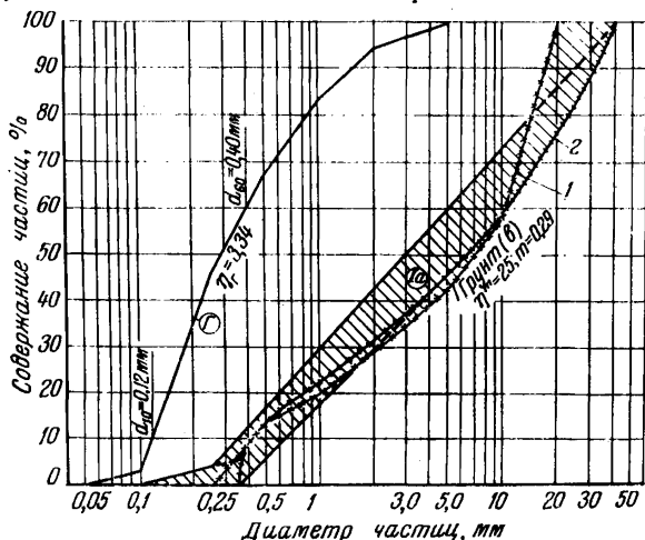
Рис. 15. График гранулометрического состава первого слоя фильтра из карьерного грунта 2
