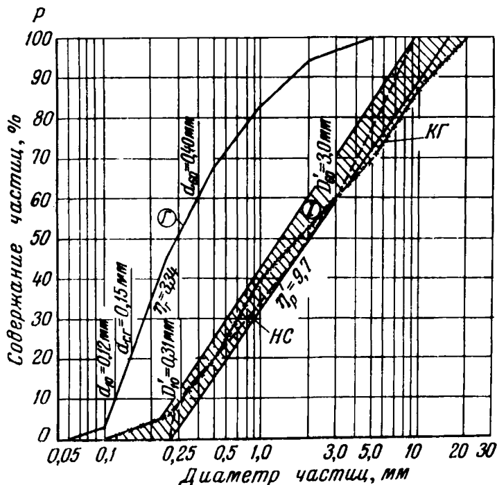
Рис. 13. График гранулометрического состава первого слоя фильтра из карьерного грунта I Г — грунт тела плиты; I — „зона допустимого гранулометрического состава грунта, пригодного для укладки в первый слой фильтра“; НС — несuffузионная кривая грунта, проходящая через точки D'_{10} и D'_{60}
