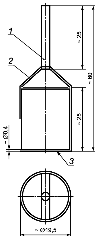
1 — штифт; 2 — поддерживающий кронштейн; 3 — кольцо
