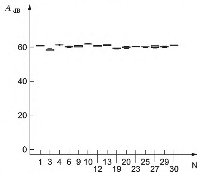
Рисунок А.2 — Отклонение результатов межлабораторных испытаний древесины
