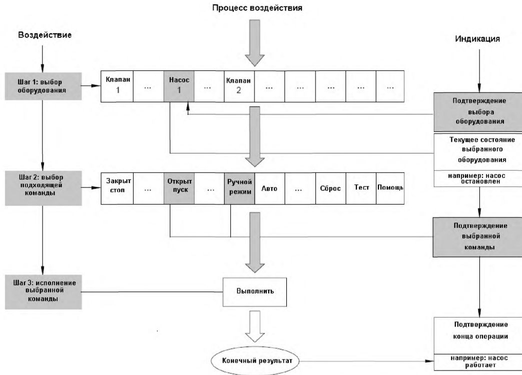
Рисунок 2 — Трехшаговая последовательность пуска для многофункционального применения
