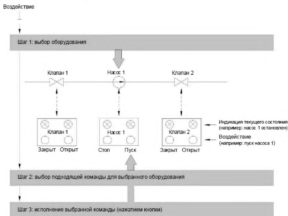
Рисунок 1 — Трехшаговая последовательность пуска для однофункционального применения
