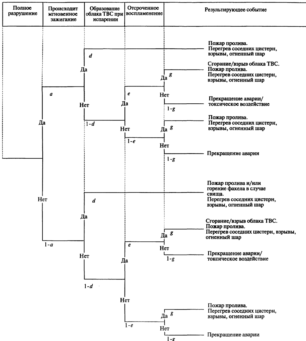
Рис. 4-5. Дерево событий для сценария с воспламенением цистерны при сливе-наливке взрывопожароопасной жидкости
