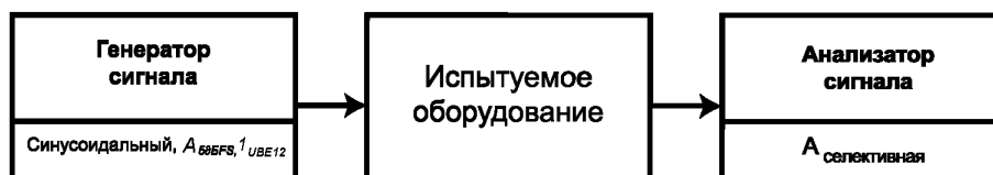
Рисунок 20 — Метод измерения собственных продуктов модуляции сигнала
