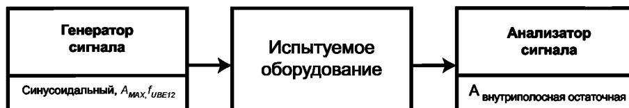
Рисунок 31 — Метод измерения восприимчивости к неустойчивой синхронизации
