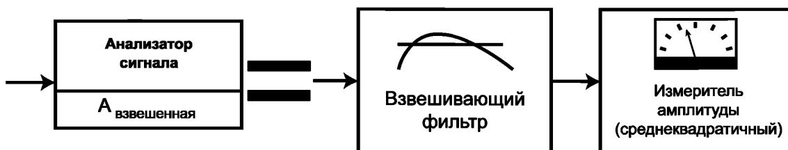
Рисунок 7 — Взвешенная амплитуда
