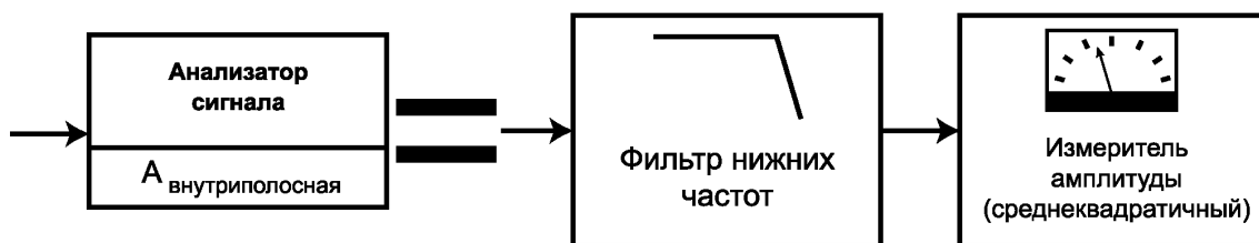
Рисунок 3 — Внутриполосная амплитуда
