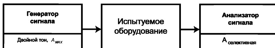
Рисунок 18 — Интермодуляционный метод
