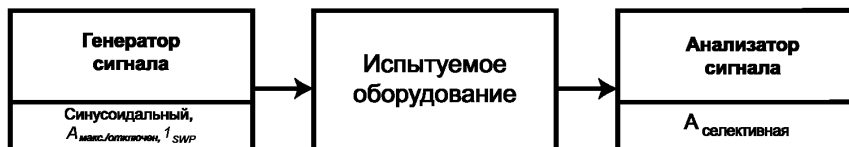
Рисунок 27 — Метод измерения нелинейных перекрестных помех
