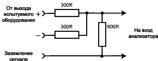
Рисунок 36 — Метод измерения баланса выходного сигнала
