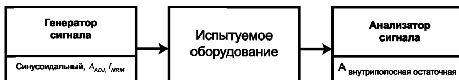
Рисунок 35 — Метод измерения полной амплитуды аналогового выходного сигнала
