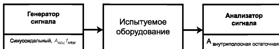
Рисунок 33 — Метод определения функционирования при перегрузке
