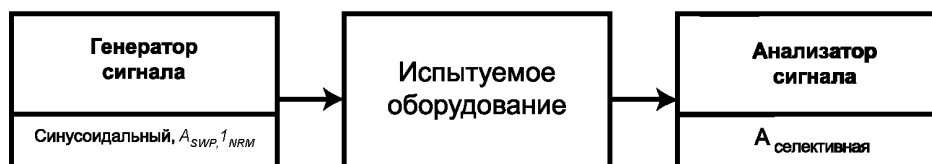
Рисунок 19 — Метод измерения амплитудно-зависимого коэффициента усиления
