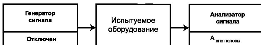
Рисунок 25 — Метод измерения отношения шумов вне полосы
