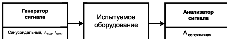
Рисунок 15 — Метод измерения общего искажения гармоник
