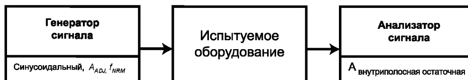
Рисунок 32 — Метод измерения полной амплитуды аналогового входного сигнала
