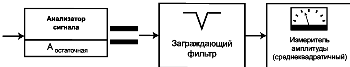
Рисунок 6 — Остаточная амплитуда
