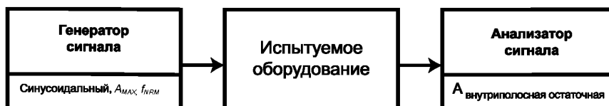
Рисунок 11 — Метод измерения искажения и шума
