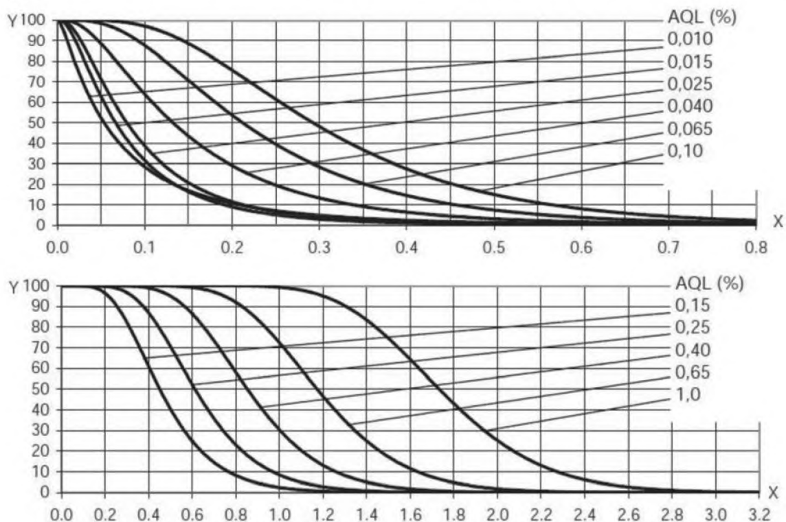
Рисунок 18 — График Q. Кривые оперативных характеристик для одноступенчатых планов выборочного контроля. Нормальный контроль
