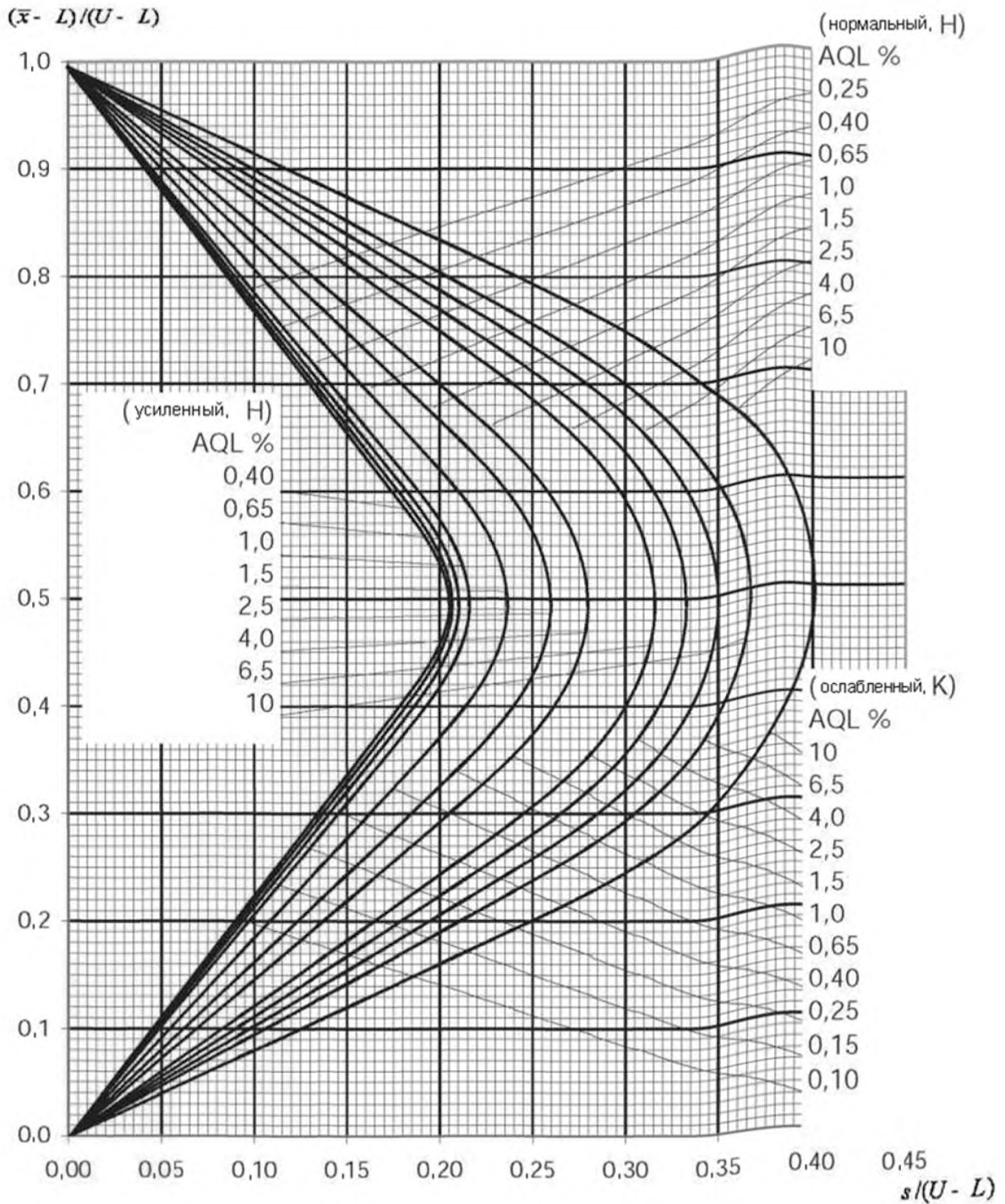
Рисунок 24 — График s-N. Приемочные кривые для объединенного контроля с двумя границами поля допуска для кода объема выборки Н при нормальном и усиленном контроле и для кода объема выборки К при ослабленном контроле
