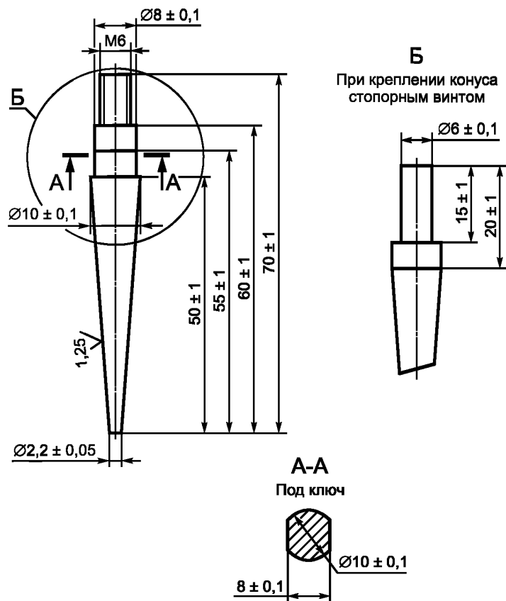
Рисунок 1 — Конус
