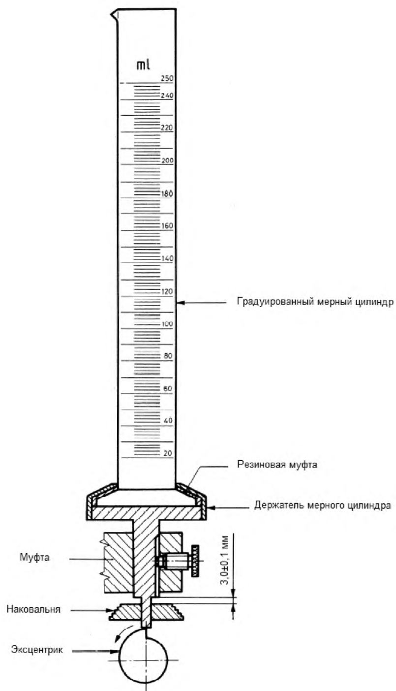
Рисунок 3 — Толчковый измеритель объема для определения насыпной плотности после уплотнения
