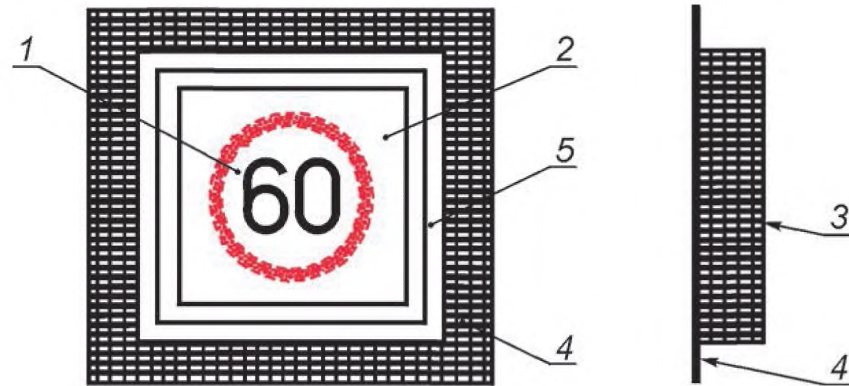
1 — изображение; 2 — поверхность отображения; 3 — направление просмотра; 4 — подложка; 5 — лицевая панель
