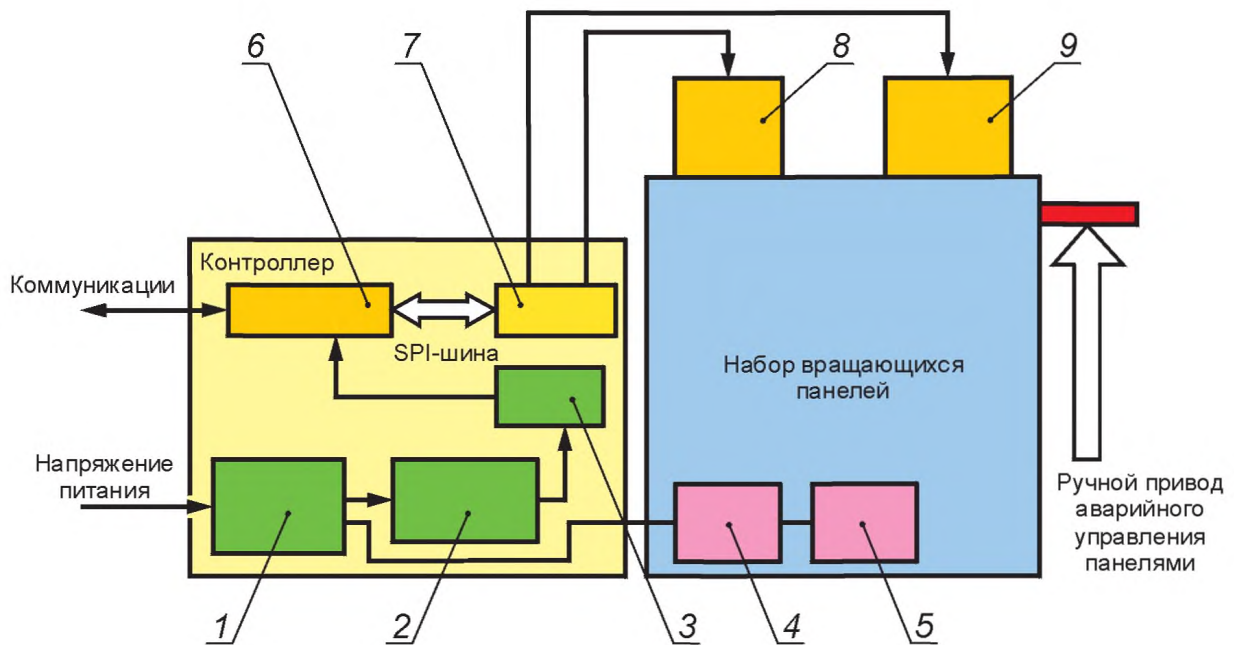
1 — электропредохранитель; 2 — трансформатор; 3 — блок питания; 4 — датчик-реле температуры; 5 — нагревательный элемент; 6 — модуль связи; 7 — модуль управления; 8 — магнитный преобразователь перемещения панелей; 9 — электромотор и механизм привода
