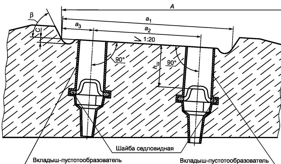
Рисунок 6, лист 1 — Подрельсовая часть шпал типа III
