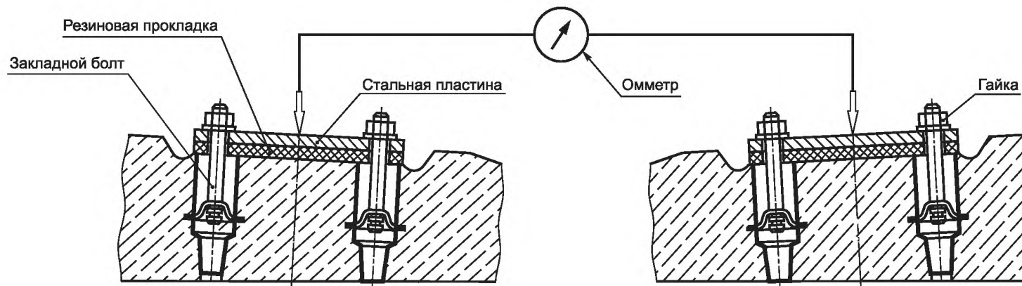
а) при болтовом скреплении
