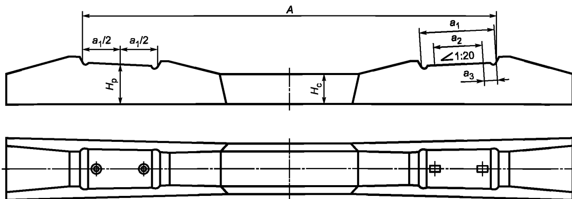
Рисунок 3 — Схема шпал типа III
