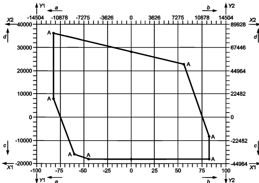
X1 — давление, МПа; X2 — давление, фунт/дюйм 2 ; Y1 — сила, даН; Y2 — сила, фунт; a — выше; b — ниже; c — сжатие; d — растяжение
