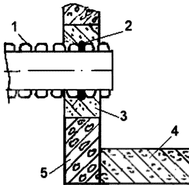
Рисунок 1 – Монтаж трубопровода наружной канализационной сети в стенку колодца
