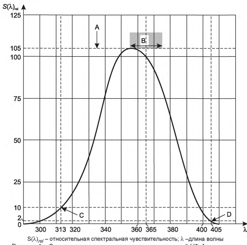
Рисунок 1 – Спектральная чувствительность измерителей УФ-А-излучения
