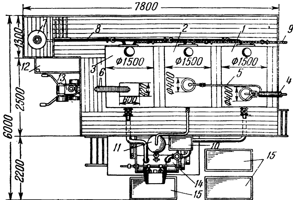
Рис. 3. Пастосмесительная установка производительностью 5 м 3 в смену на огневом обогреве (Углеметаллургстрой)
