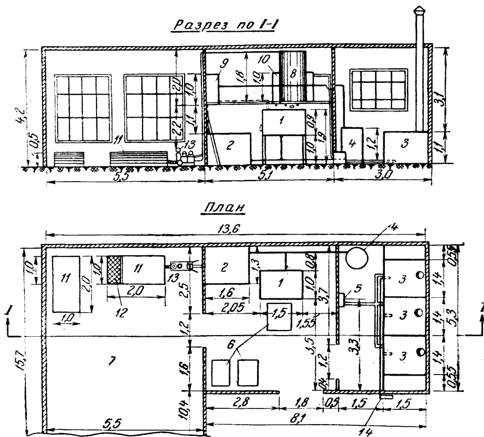
Рис. 29. Пастосмесительная установка производительностью 4 т в смену на паровом нагреве (Ленотделстрой-2)
