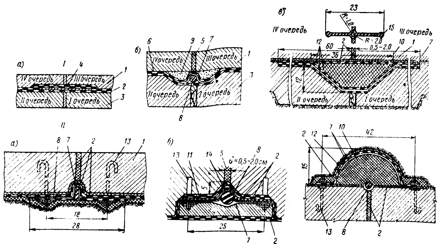
Рис. 11. Устройство пересечений холодной асфальтовой гидроизоляции с деформационными швами
