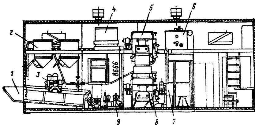
Рис. 32. Разрез по контейнеру пастосмесительной установки МД-96
