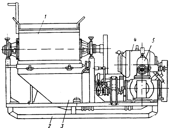
Рис. 36. Растворосмесительный агрегат С-362
