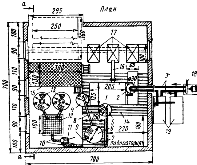
Рис. 28. Пастосмесительная установка производительностью 8—10 т в смену (большая установка ВНИИГа)
