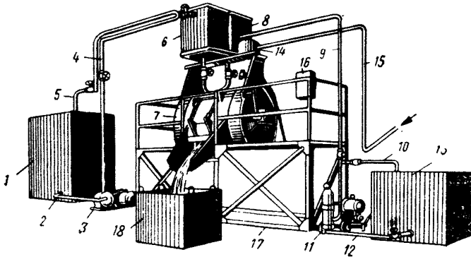
Рис. 3. Принципиальная схема пастосмесительной установки 1—битумный котел; 2, 4 и 5—битумопровод; 3—битумный насос; 6—дозатор битума; 7—мешалка-пастосмеситель; 8—дозатор эмульгатора; 9—10—12—растворопроводы; 11—растворонасос; 13—емкость для эмульгатора; 14—дозатор воды; 15—водопровод; 16—электрощит; 17—помост; 18—емкость для готовой пасты.
