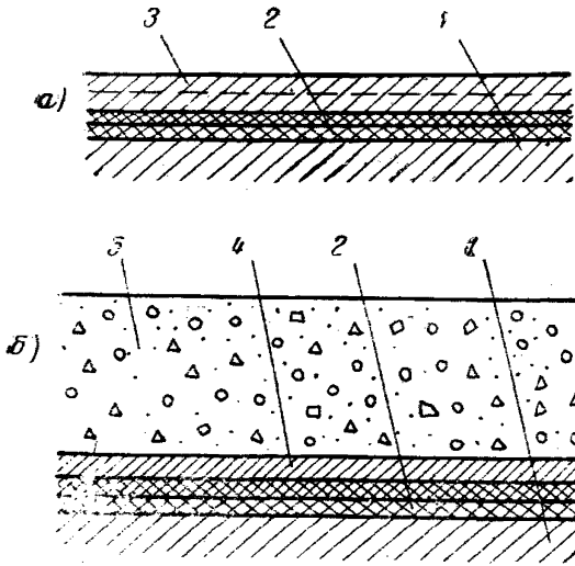
Рис. 7. Конструкция холодной асфальтовой гидроизоляции на перекрытиях
