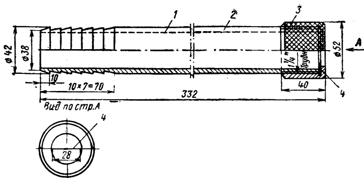
Рис. 35. Бескомпрессорная форсунка
