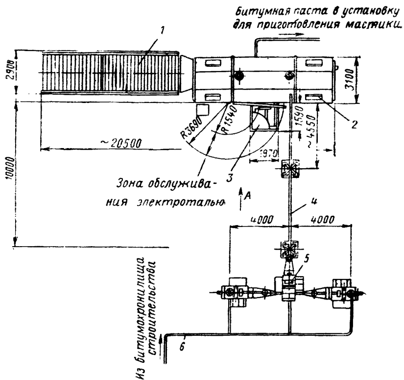
Рис. 31. План пастосмесительной установки МД-96 Ленфилиала Оргэнергостроя производительностью 10 т в смену 1—известковая яма; 2—пастосмесительная установка; 3—емкость с готовой битумной пастой; 4—циркуляционный битумопровод; 5—битумоплавильные котлы Д-385; 6—подача битума от битумохранилища.
