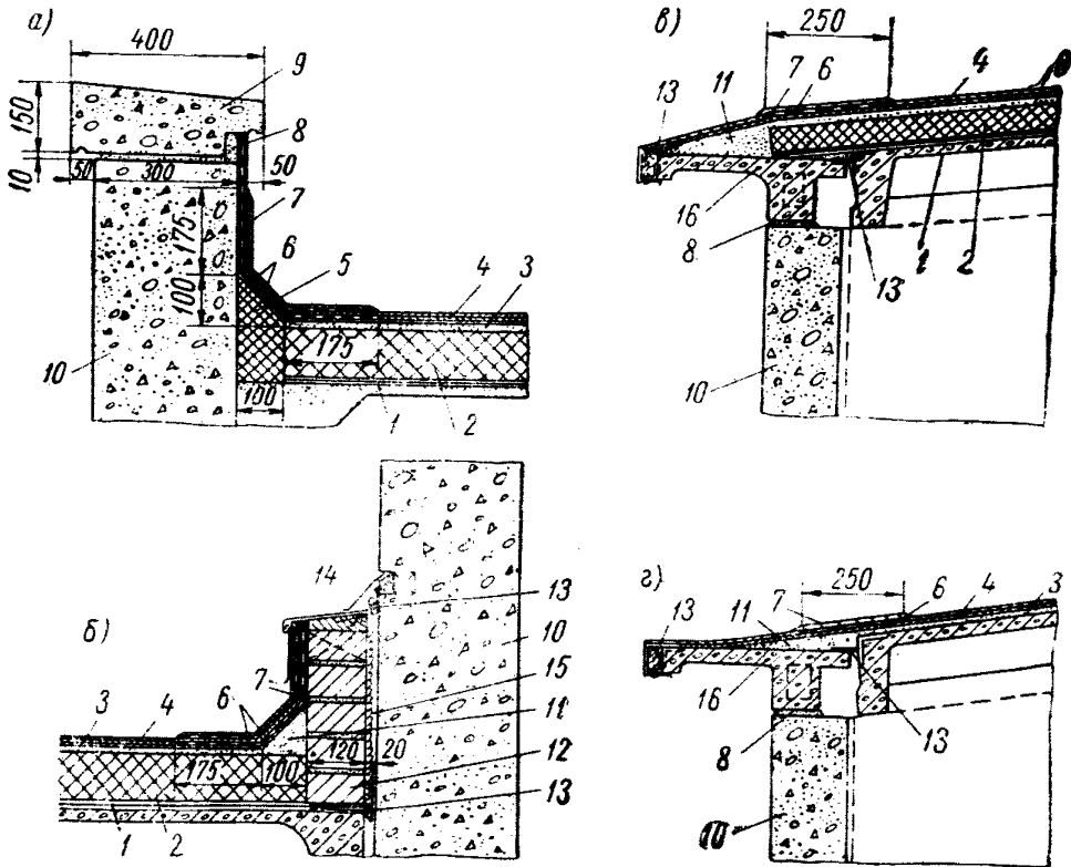
Рис. 15. Детали сопряжений безрулонной кровли с парапетом, стеной и карнизными свесами
