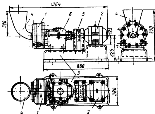
Рис. 23. Диспергатор Гипростроммаша
