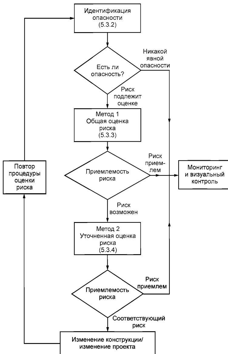
Рисунок 1 — Система экспертной оценки риска
