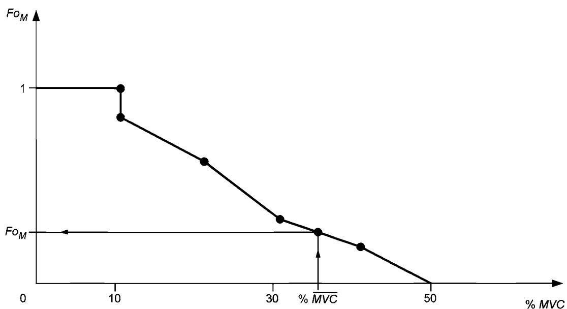
Рисунок С.2 — Определение значения F_{oM} (этап 7)
