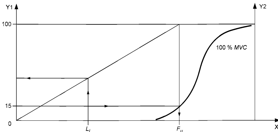
Рисунок С.1 — Определение величины \% MVC_i (этапы 1–5)
