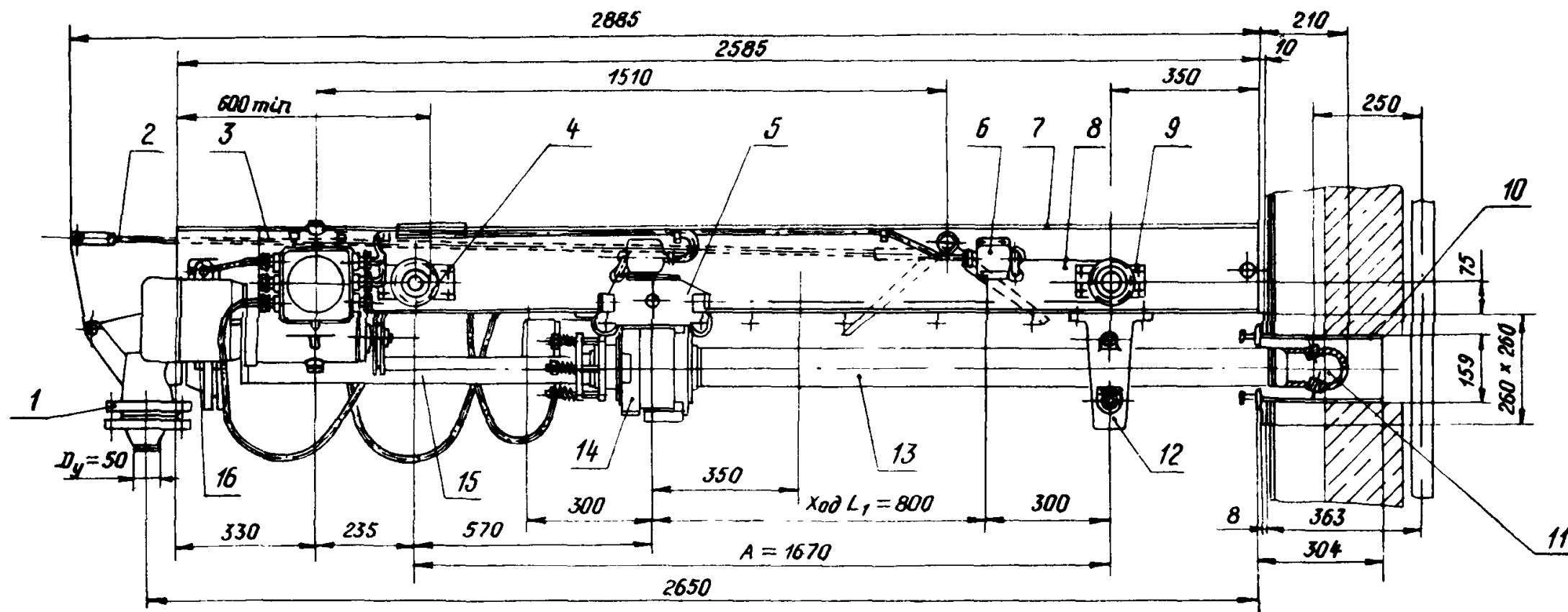
1 — узел клапана; 2 — рычажный механизм; 3 — редуктор; 4 — промежуточная передача; 5 — каретка; 6 — проводка кабелей; 7 — балка; 8 — цепь приводная; 9 — узел звездочки. 10 — закладная втулка; 11 — сопловая головка; 12 — подшипник передний; 13 — обдувочная труба; 14 — редуктор; 15 — труба подводящая с фланцем; 16 — кронштейн Черт. 3
