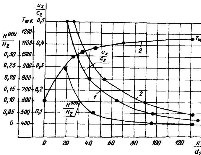
1 — для изотермической струи; 2 — для неизотермической струи T_n=600 К; T_r=1200 К; a=0,05
