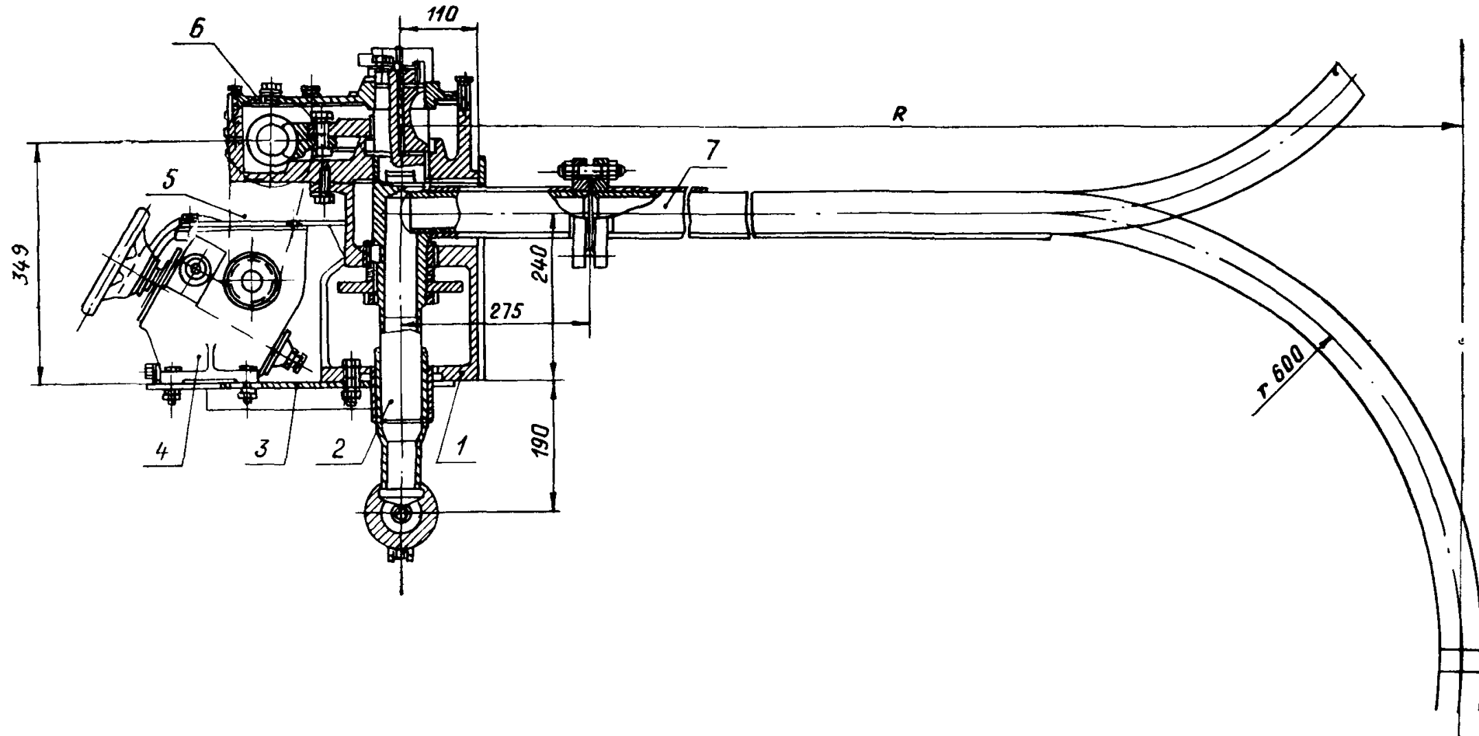
1 — корпус; 2 — труба осевая; 3 — плата; 4 — привод; 5 — цепная передача; 6 — редуктор; 7 — обдувочная труба Черт. 6
