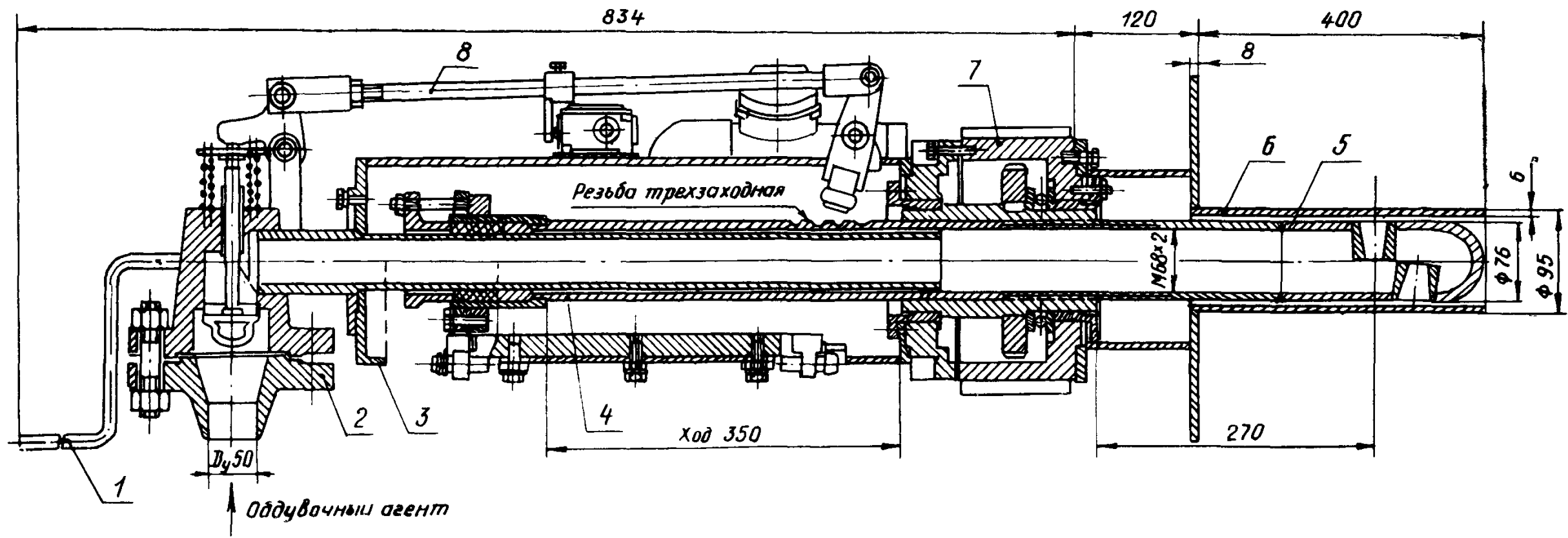
1 — рукоятка; 2 — клапан; 3 — корпус; 4 — шпindelь; 5 — сопловая головка; 6 — втулка закладная; 7 — редуктор; 8 — рычажный механизм Черт. 2
