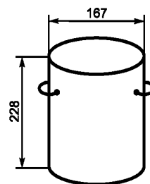
Рисунок 2 — Измерительный контейнер (малый)
