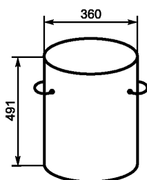
Рисунок 1 — Измерительный контейнер (большой)
