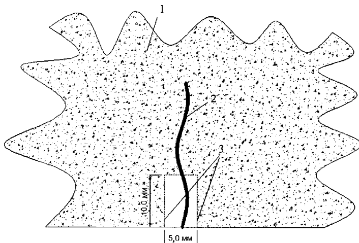
1 – тело бетона; 2 – трещина; 3 – линии разделки трещины Рисунок 2 – Схема подготовки трещин при гидрозащите
