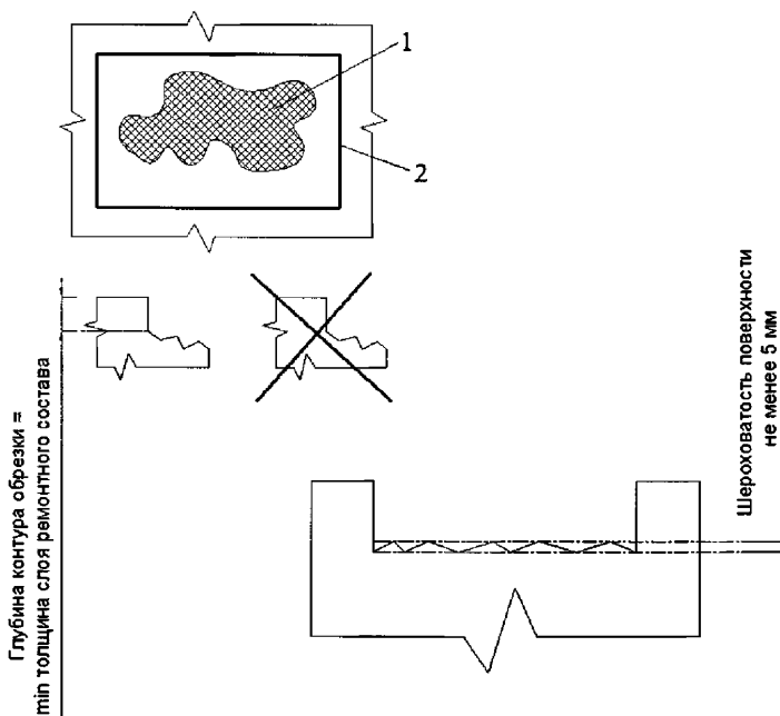
Рисунок 3 – Подготовка ремонтных зон
