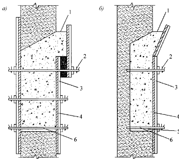
а) – двухсторонняя опалубка; б) – односторонняя опалубка
