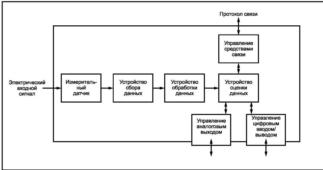
Рисунок 1 — Структура преобразователя
