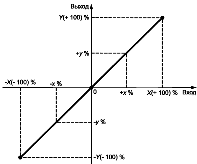
Рисунок 2 — Кривые передаточной функции
