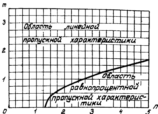
Рис.16. График для определения типа пропускной характеристики РО, управляющего параллельным потоком жидкости
