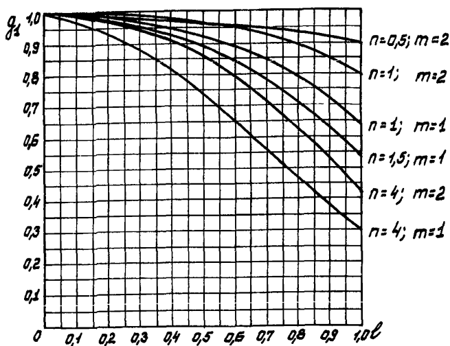
Рис. 9. Графики рабочих расходных характеристик для ветви с технологическим оборудованием (схема 2, РО с равнопроцентной пропускной характеристикой)
