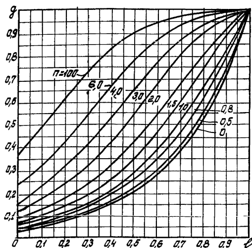
Рис. 4 Графики рабочих расходных характеристик РО с равнопроцентной пропускной характеристикой, установленного на регулируемом участке по схеме I
