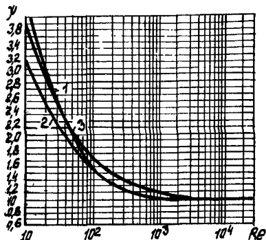
Рис. I Зависимость \psi от числа Рейнольдса.
