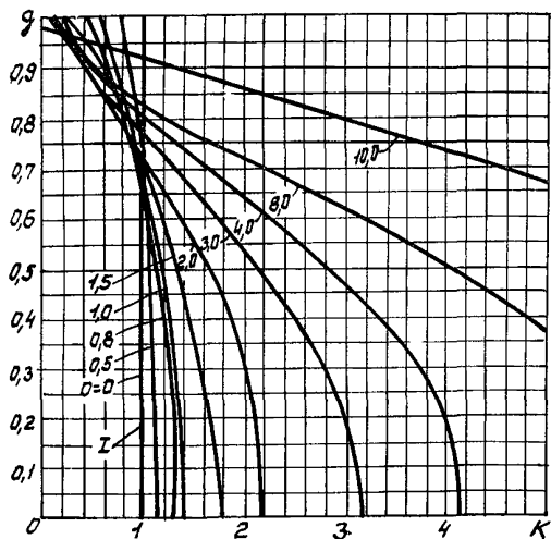
Рис. 5 Графики зависимости относительного расхода q от коэффициента передачи K для РО с линейной пропускной характеристикой, установленного на регулируемом участке по схеме I
