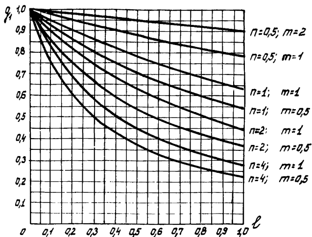
Рис.8. Графики рабочих расходных характеристик для ветви с технологическим оборудованием (схема 2, P0 с линейной пропускной характеристикой)
