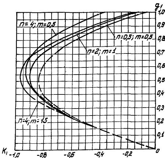
Рис. II Графики зависимости Q_1 = f(K_1) для РО с равнопроцентной пропускной характеристикой.
