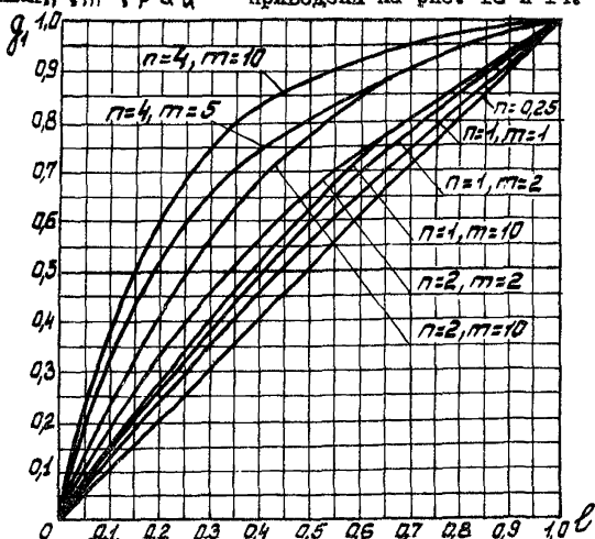
Рис. 13. Рабочая расходная характеристика трехходового РО с равновеликими окнами ( a = 1 , \rho = \infty )
