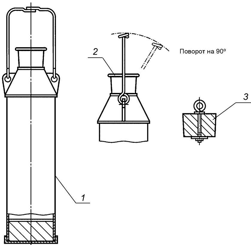
1 — цилиндрический контейнер из нержавеющей стали; 2 — конусообразная горловина; 3 — пробка
