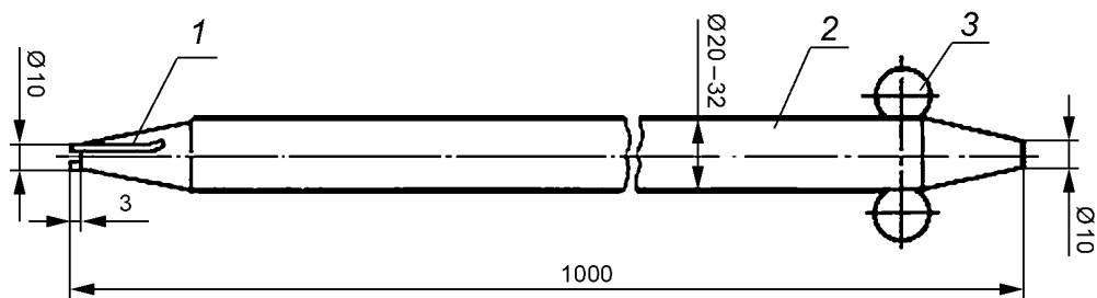
1 — ножка; 2 — трубка; 3 — ушко
