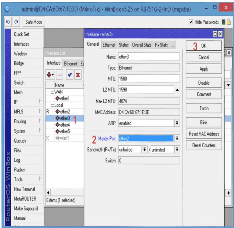
Рис. В.11. Объединение портов ether2 – ether3 в свитч.
