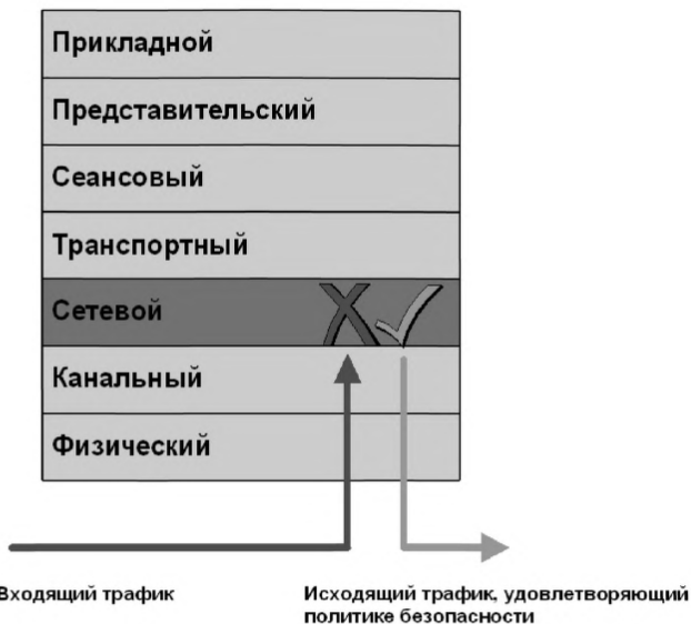
Рис. 4.3. Место пакетного фильтра в модели OSI
