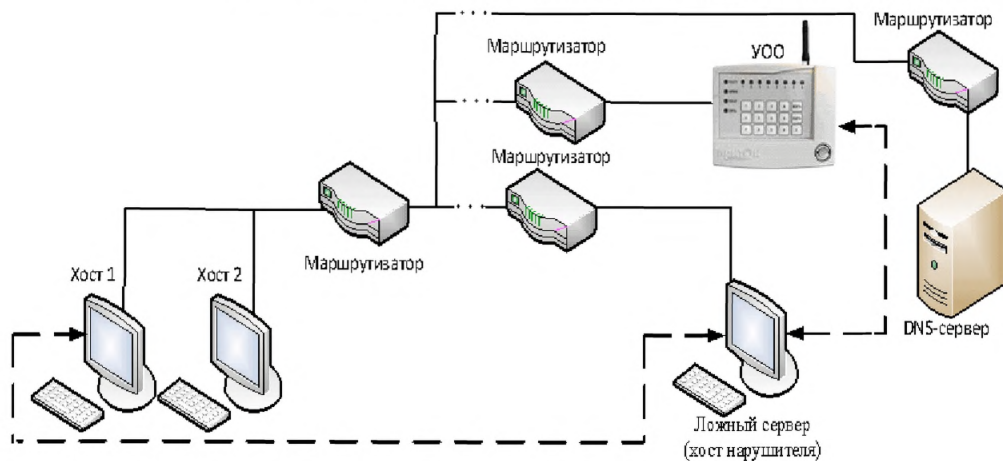
Рисунок 3.8. Схема реализации угрозы «внедрение ложного DNS-сервера» путем шторма DNS-ответов на компьютер сети
