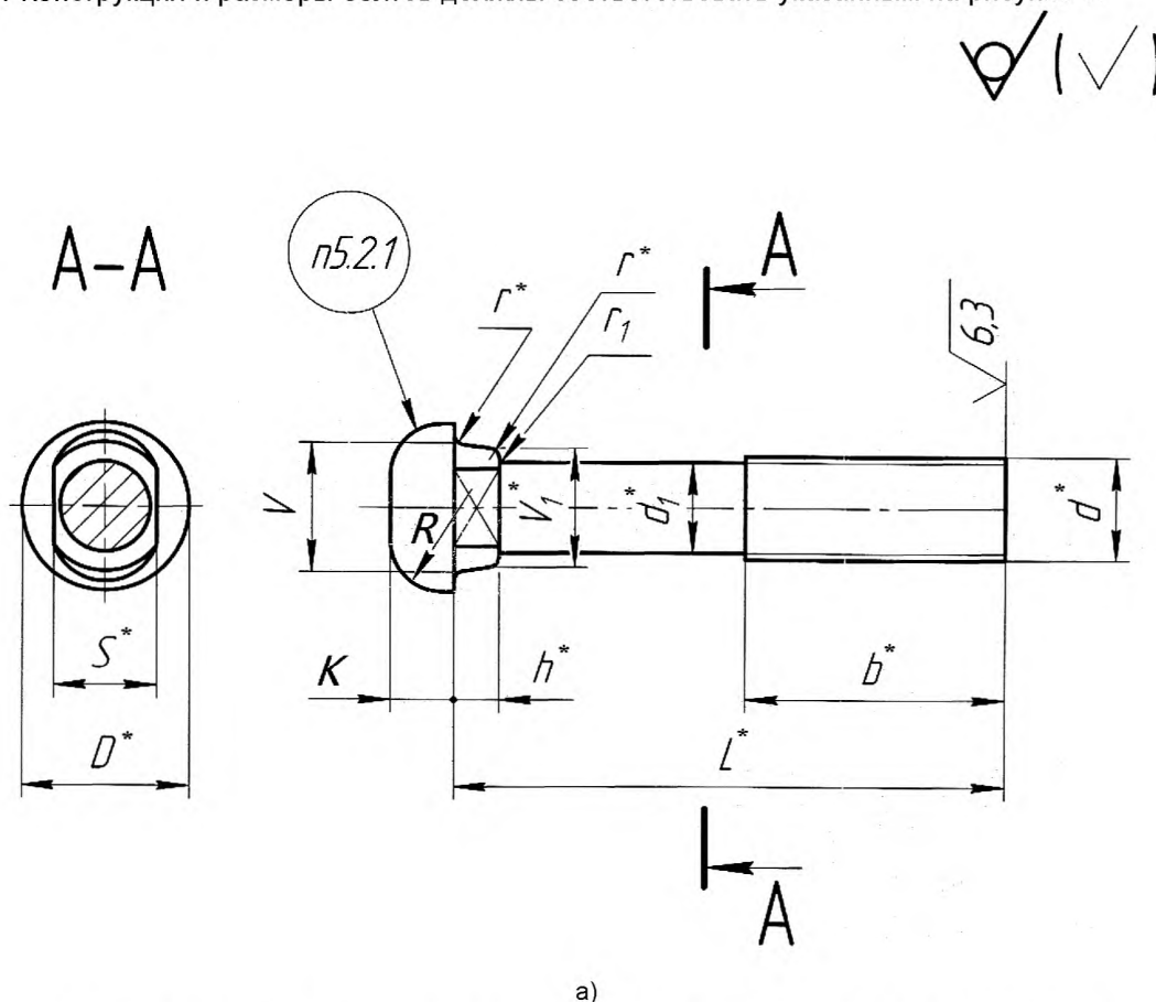
Рисунок 1, лист 1 — Конструкция и размеры болтов: а) исполнение 1; б) исполнение 2
