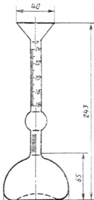
Рисунок 1 — Прибор Ле-Шателье
