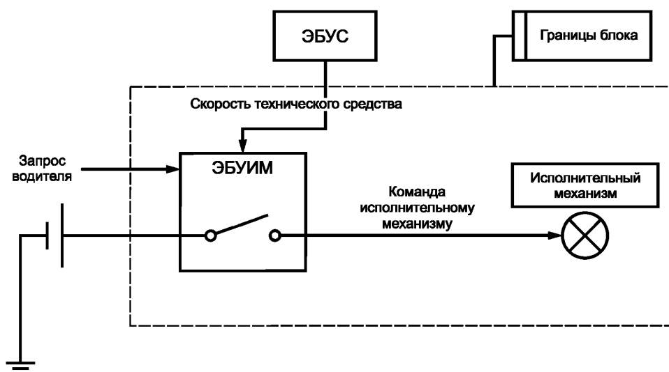
Рисунок 22 — Границы устройства
