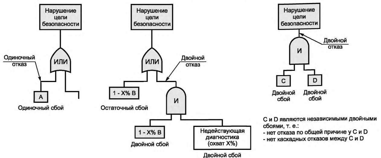
Рисунок В.4 — Примеры FTA для одиночного, остаточного и двойного сбоев
