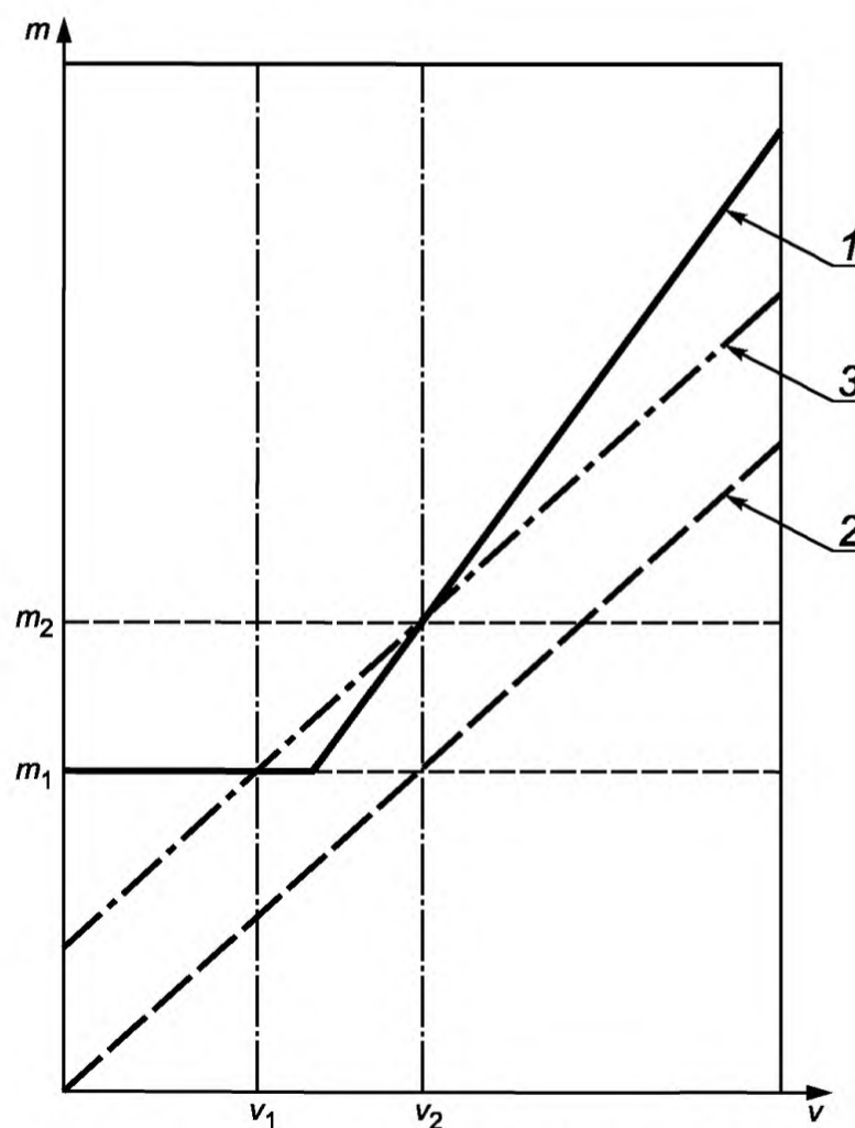
1 — связанная с безопасностью нижняя граница \mu_{SafRel, A, min} датчика A_Master; 2 — возвращаемое значение идеального датчика с нулевым допуском (как эталон); 3 — наихудший случай порога обнаружения \mu_{A, Master, wc} .
