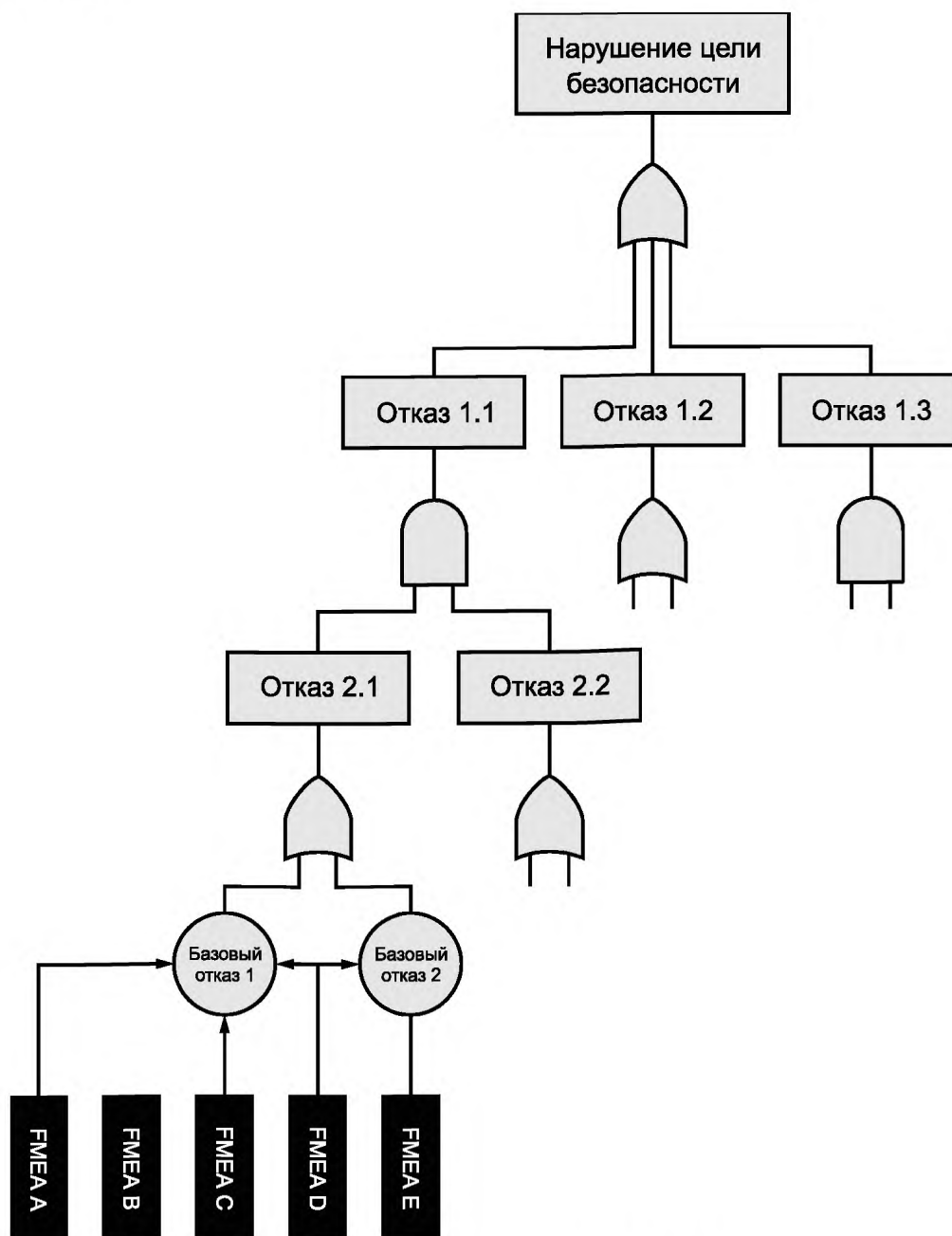
Рисунок В.3 — Объединение FTA и FMEA
