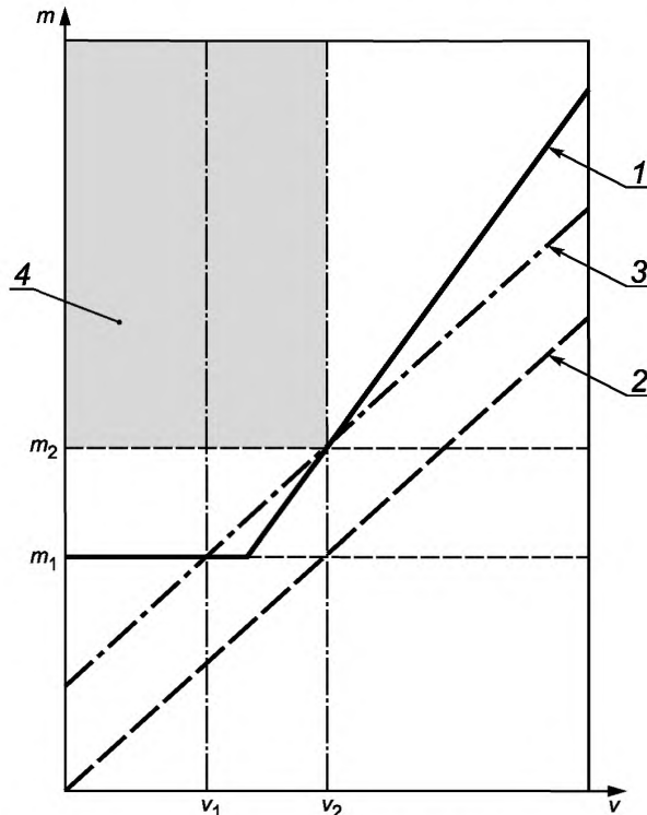
1 — связанная с безопасностью нижняя граница \mu_{\text{SafRel},A,\text{min}} датчика A_Master; 2 — возвращаемое значение идеального датчика с нулевым допуском (как эталон); 3 — наихудший случай порога обнаружения \mu_{A\_Master,wc} ; 4 — двойные обнаруживаемые сбои
