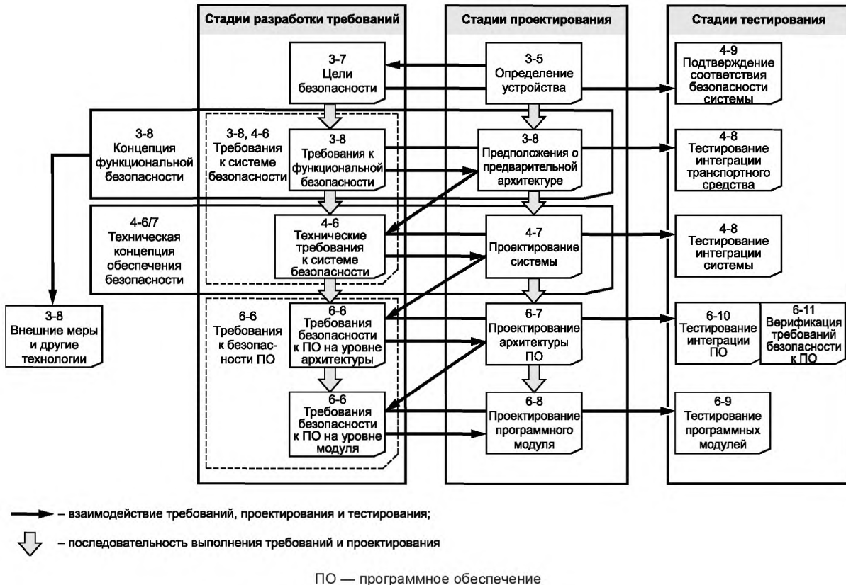
Рисунок 8 — Начинаящая от формирования концепции последовательность разработки требований безопасности, проектирования и тестирования для программного обеспечения
