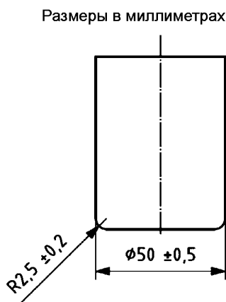
Рисунок 1 — Схема штампа
