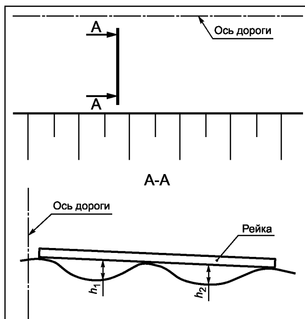
Рисунок 1 — Схема проведения измерений величины колеи
