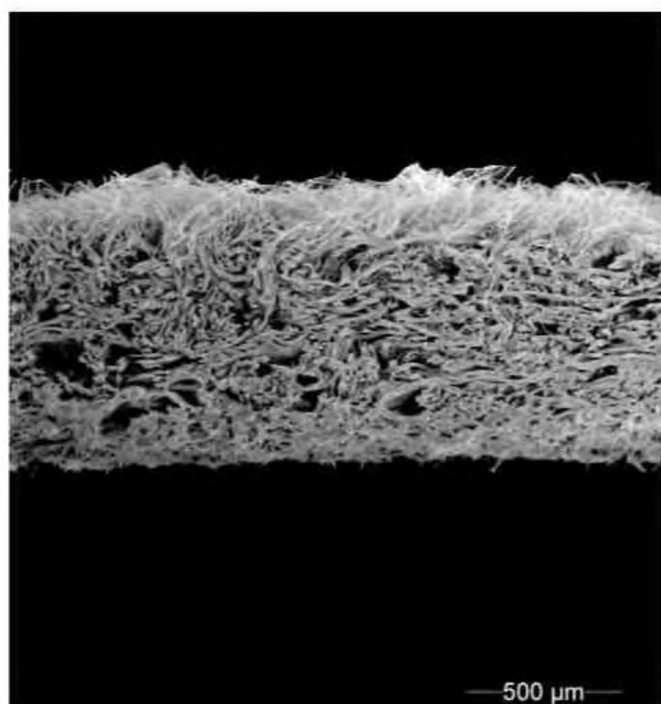
а) Сечение материала микрофибра при небольшом увеличении
