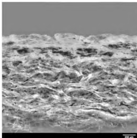
Рисунок В.2 — Типичное сечение шеврета
