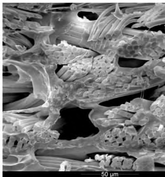
б) Сечение материала микрофибра при большом увеличении
