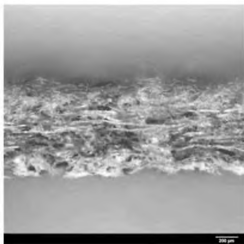
Рисунок В.7 — Типичное сечение материала микрофибра
