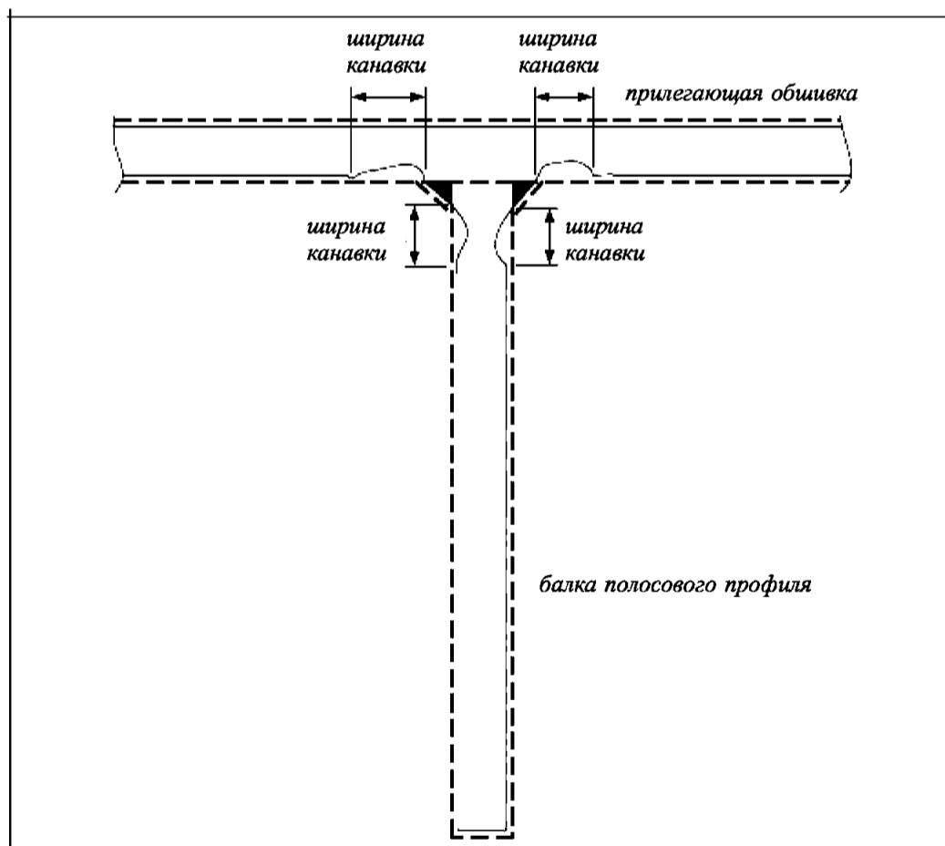
Рис. 1.2.1-4 Канавочный износ
