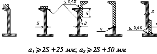
Рис. 5.2.4.1-1 Подкрепление балок набора:
