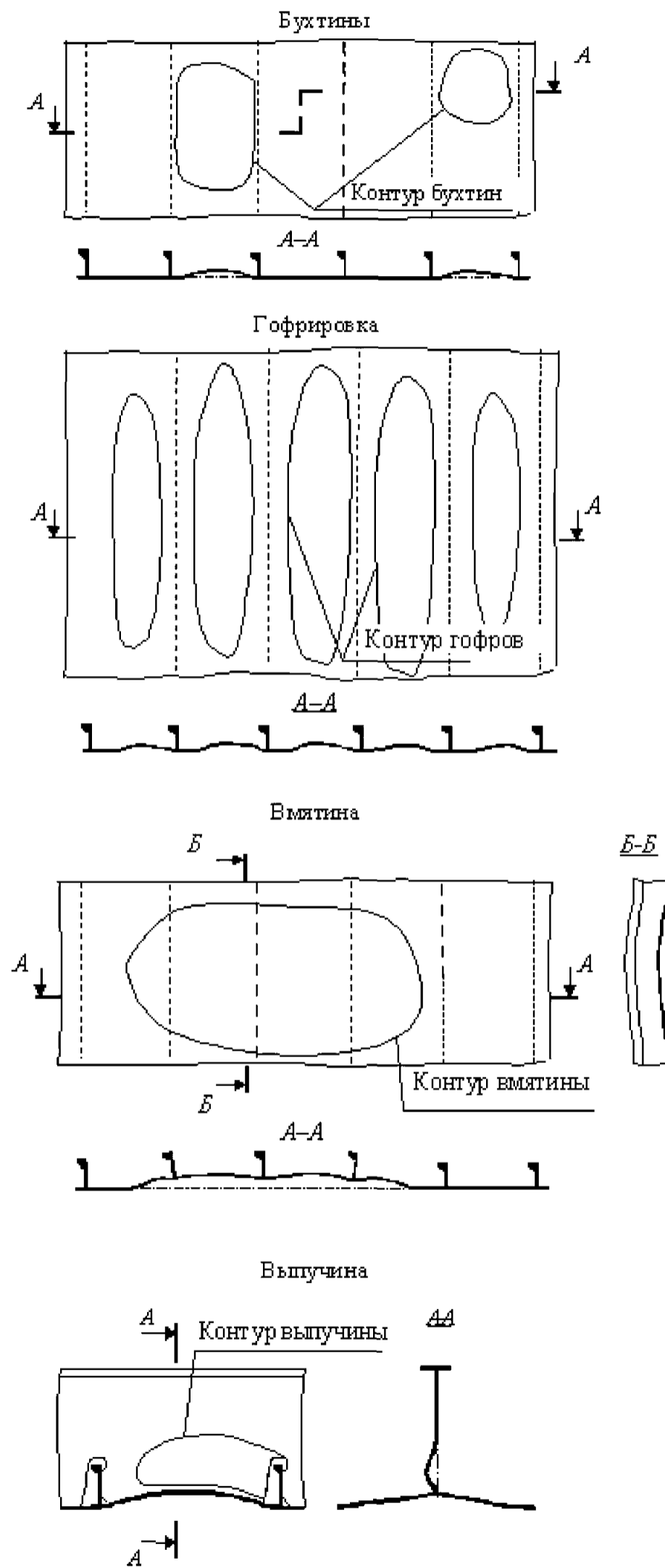
Рис. 1.2.1-1 Виды остаточных деформаций
