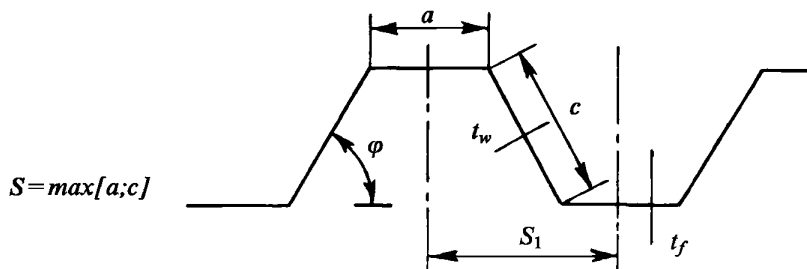
Рис. 5.9.2.3.1.1 Схема поперечной гофрированной переборки
