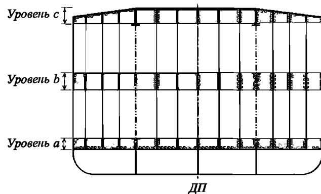
Рис. 7.2.3.4 Уровни а, b и с детального освидетельствования поперечной переборки грузового трюма, не имеющего твиндек, на судах, предназначенных для перевозки сухих генеральных грузов
