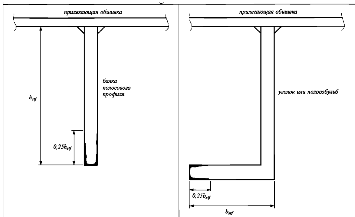
Рис. 1.2.1-5 Коррозия кромок
