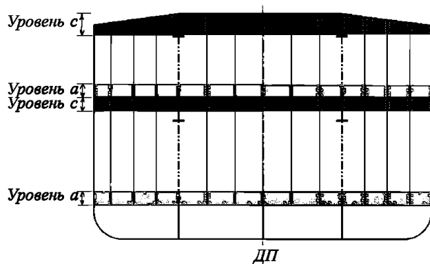
Рис. 7.2.3.3 Уровни а и с детального освидетельствования поперечной переборки твиндечного грузового трюма на судах, предназначенных для перевозки сухих генеральных грузов
