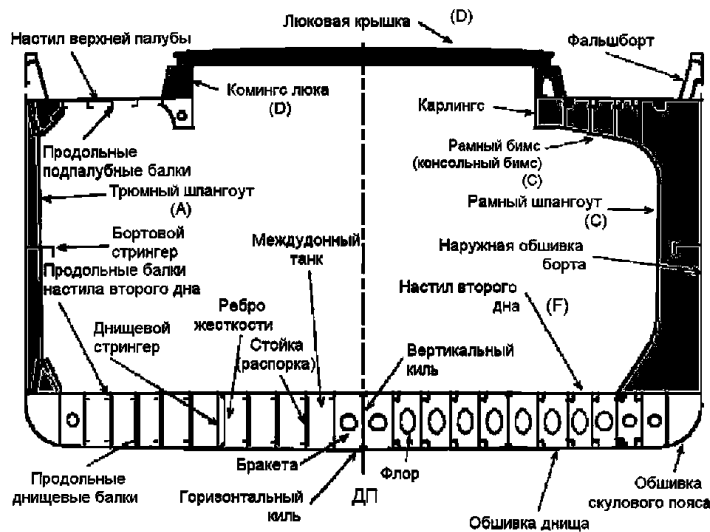
Рис. 7.2.3.2 Районы А, С, D и F детального освидетельствования судов, предназначенных для перевозки сухих генеральных грузов
