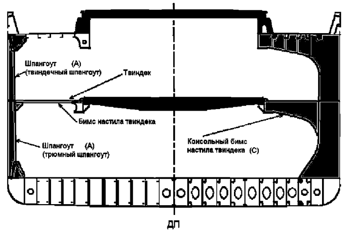
Рис. 7.2.3.2 Районы А, С, D и F детального освидетельствования судов, предназначенных для перевозки сухих генеральных грузов
