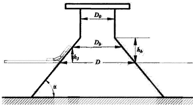
Рис. 3.3.2.3.18-1 Платформа с расширяющимися вниз коническими бортами
