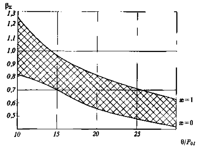
Рис. 3.1.6.1 Обобщенный коэффициент динамичности: \theta — несущая частота акселерограммы; P_{01} — низшая частота горизонтальных колебаний
