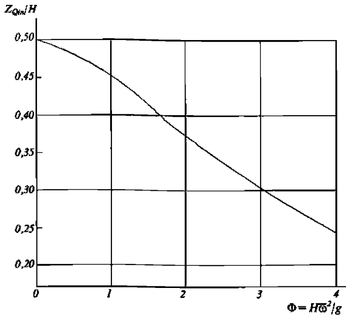
Рис. 3.1.4.13-3 Зависимость Z_{Qin}/H от параметра \Phi = H\omega^2/g
