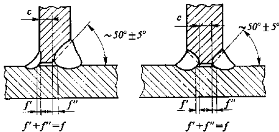
Рис. 2.6.4.1 Примеры двухсторонних тавровых соединений с конструктивным непроваром
