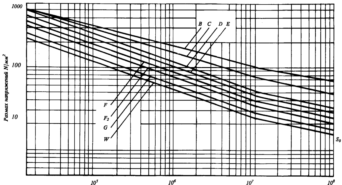
Рис. 2.4.4.8-1 Кривые усталости
