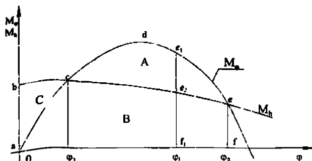
Рис. 3.1.1-2 Диаграмма статической устойчивости без учета качки
