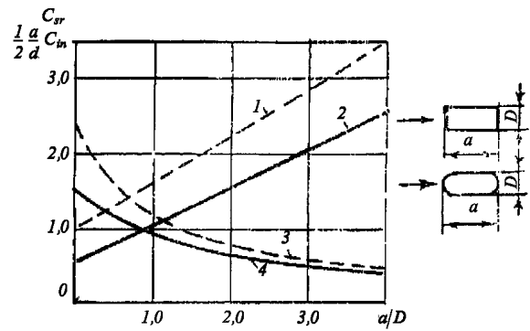
Рис. 3.1.4.1 Коэффициенты скоростного C_{sr} (3, 4) и инерционного C_{in} (1, 2) сопротивления сечений: ————— эллиптических (круглых a/D=1 ); - - - - - прямоугольных
