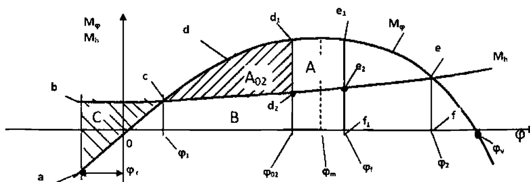
Рис. 3.1.1-1 Диаграмма статической устойчивости с учетом качки:
