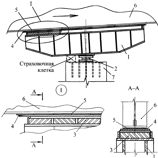
1 – накаточная (балансирующая) балка; 2 – опорная часть (шарнир); 3 – резиновая прокладка; 4 – контртело (стальной полированный лист); 5 – полимерные прокладки (карточки скольжения); 6 – надвигаемая конструкция; 7 – подферменный опоры
