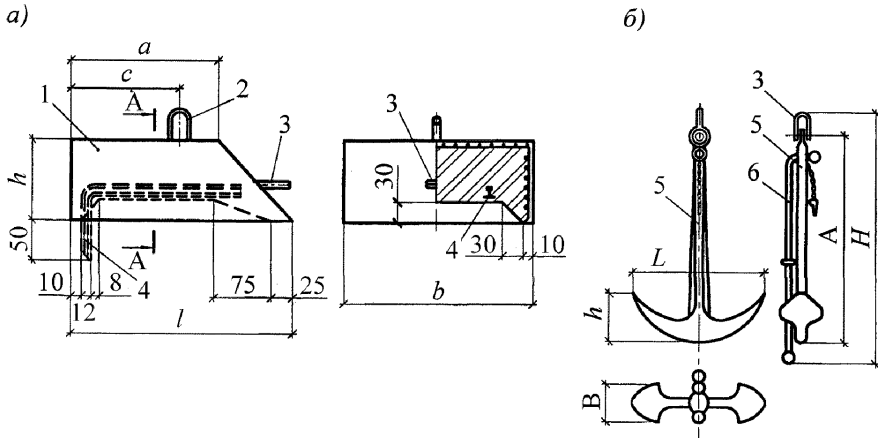
Рисунок 5.22 – Схема якорного закрепления плавсредства
