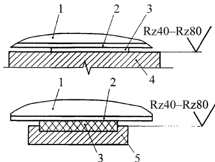
Рисунок 5.12 – Устройство скольжения циклического действия
