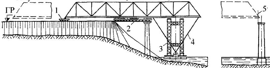
1 – каретка с балансиром; 2 – накаточные пути и катки; 3 – плавучая опора; 4 – стальные канаты; 5 – конечное положение пролетного строения
