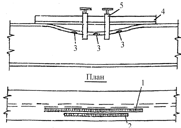
1, 2 – продольные полосы нагрева для правки грибовидности; 3 – поперечные полосы для правки волнистости по кромке; 4 – уголок; 5 – струбцины винтовые Рисунок И.14 – Термомеханическая правка деформации типа односторонней грибовидности и волнистости по кромке
