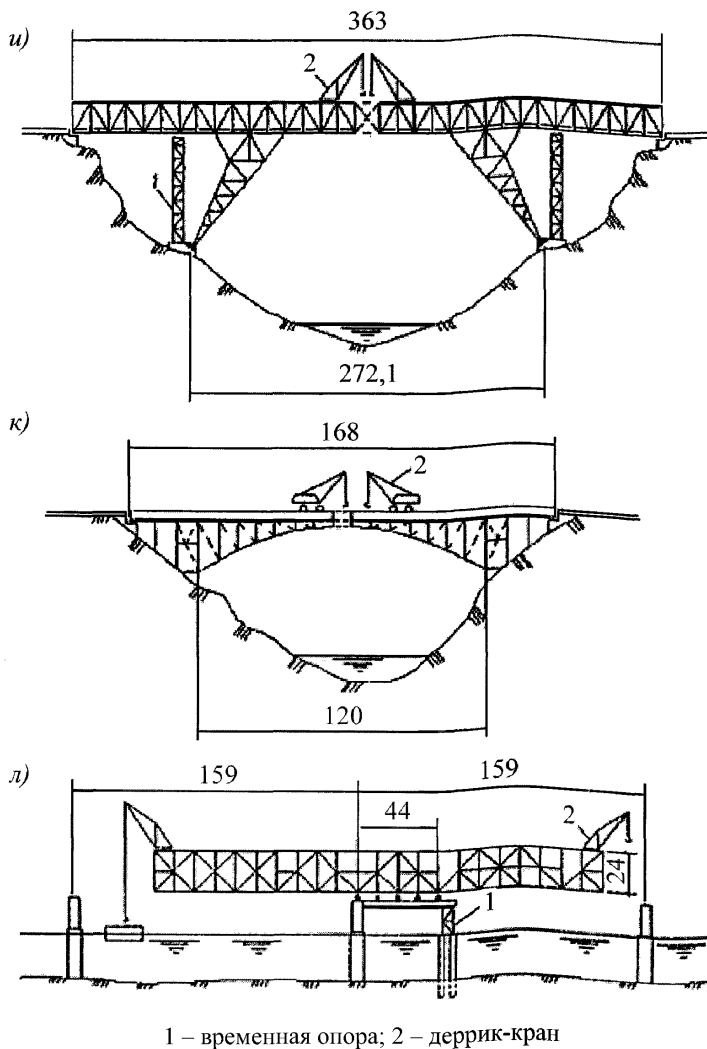
Рисунок 6.15 – Схемы монтажа решетчатых пролетных строений
