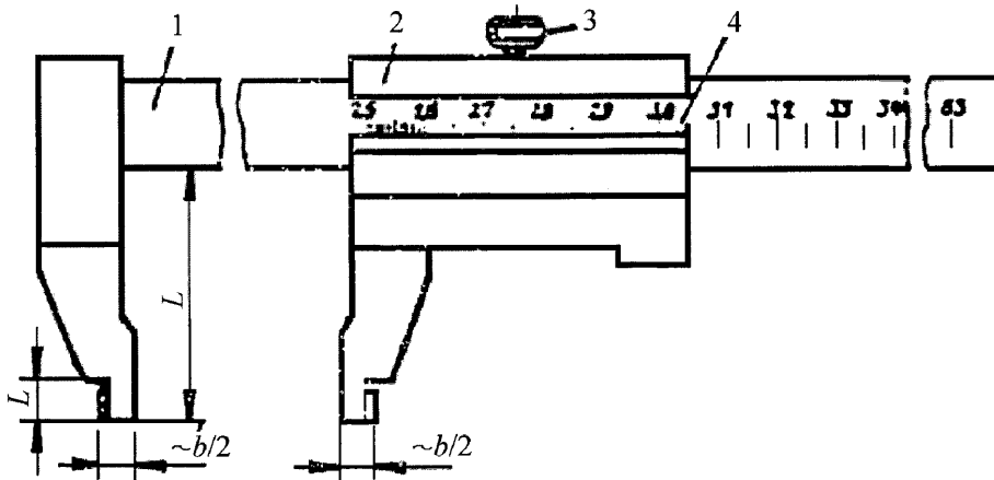
Рисунок Г.1 – Штангенциркуль ШЦ-II с точностью отсчета по нониусу 0,05 мм
