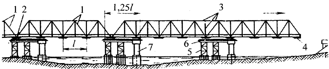
Рисунок 5.9 – Схема накаточных путей для надвигки на катках
