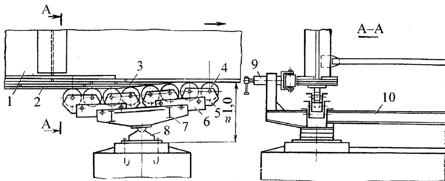
1 – пролетное строение; 2 – переходной мостик; 3 – прокладки; 4 – ролик; 5 – малый балансир; 6 – средний балансир; 7 – главный балансир; 8 – опорная часть картки; 9 – направляющее устройство; 10 – соединительная рама
