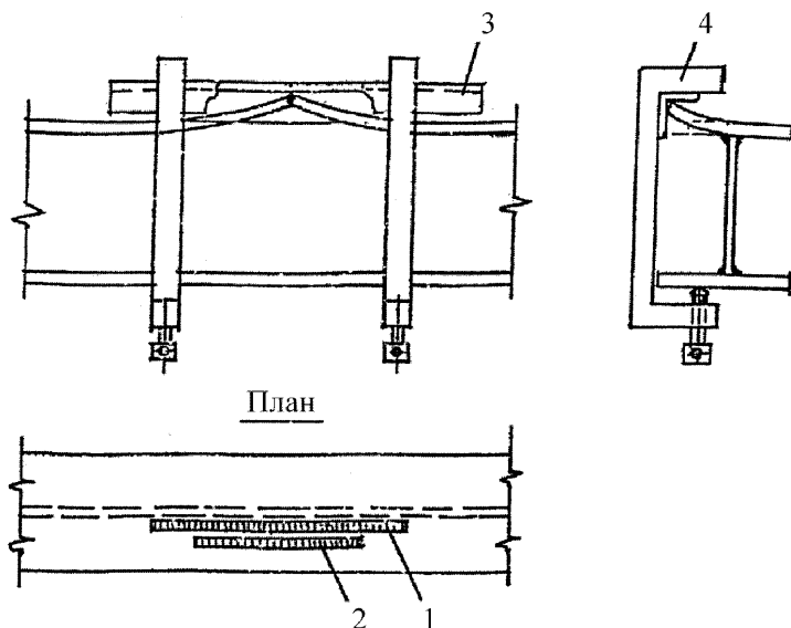
1, 2 – полосы нагрева; 3 – уголок; 4 – струбцины
