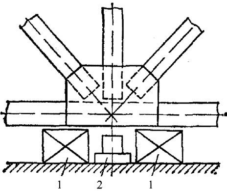
Рисунок 6.2 – Узел опирания фермы пролетного строения на подмости
