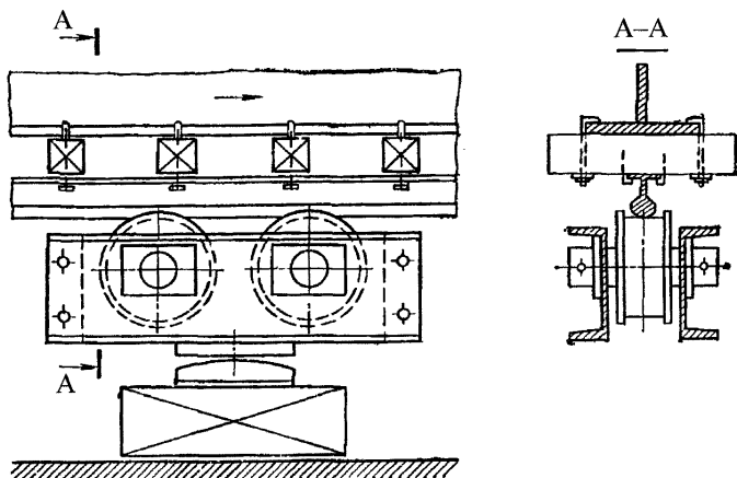
Рисунок 5.3 – Картки для продольной навигации пролетного строения по верхнему накаточному пути
