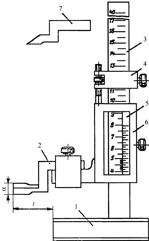
1 – основание; 2 – измерительная ножка; 3 – штанга; 4 – микрометрическая подача; 5 – нониус; 6 – рамка; 7 – разметочная ножка Рисунок Г.4 – Штангенрейсмас
