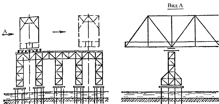
Рисунок 6.12 – Схема поперечной перекатки пролетного строения по пирсам
