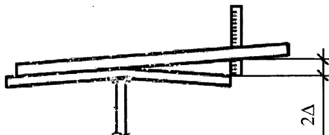
Рисунок Г.17 – Измерение симметричной грибовидности линейками
