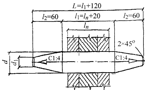
Рисунок 6.26 – Конструкция пробки
