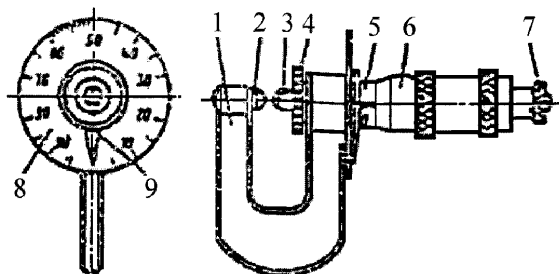
1 – скоба; 2 – пятка; 3 – микрометрический винт; 4 – стопор; 5 – стембель; 6 – барабан; 7 – трещотка (фрикцион); 8 – циферблат; 9 – стрелка
