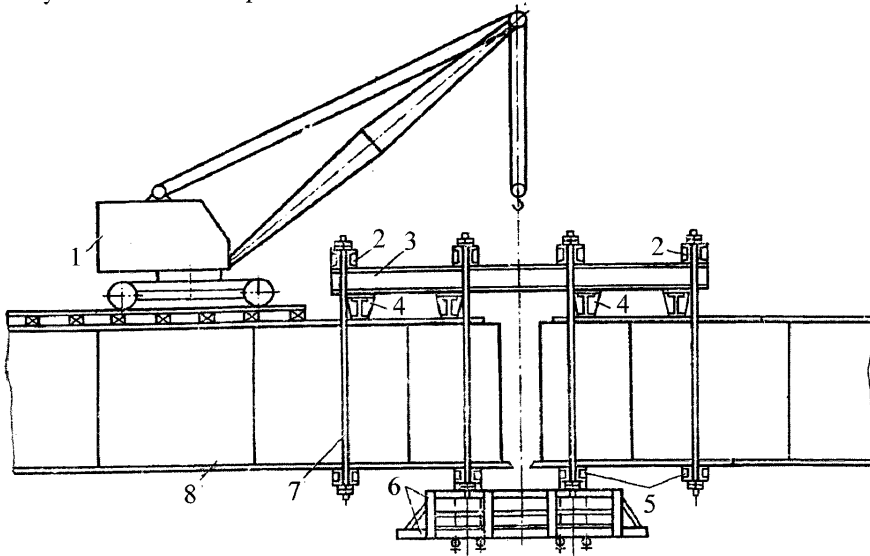
1 – монтажный кран; 2 – верхние поперечные пакеты; 3 – продольные пакеты; 4 – опорная балка; 5 – нижние поперечные пакеты; 6 – подмости; 7 – тязи; 8 – пролетное строение
