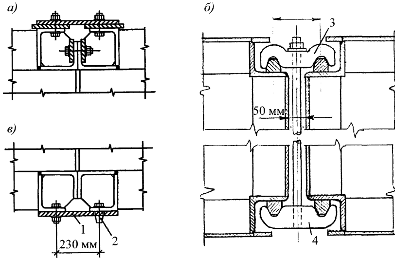
а) – болтовой стык; б) – вариант сцena для сборки на плаву; в) – замковый стык; 1 – стыковая планка; 2 – конический самозахватный штырь; 3 – верхний замок; 4 – штанга
