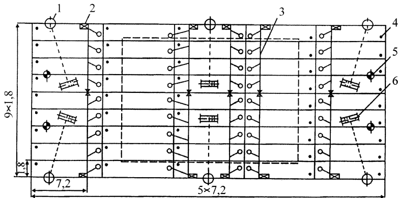
1 – кирпичная планка; 2 – водяной насос; 3 – разводящая сеть; 4 – открытые отверстия; 5 – рым; 6 – ручная лебедка
