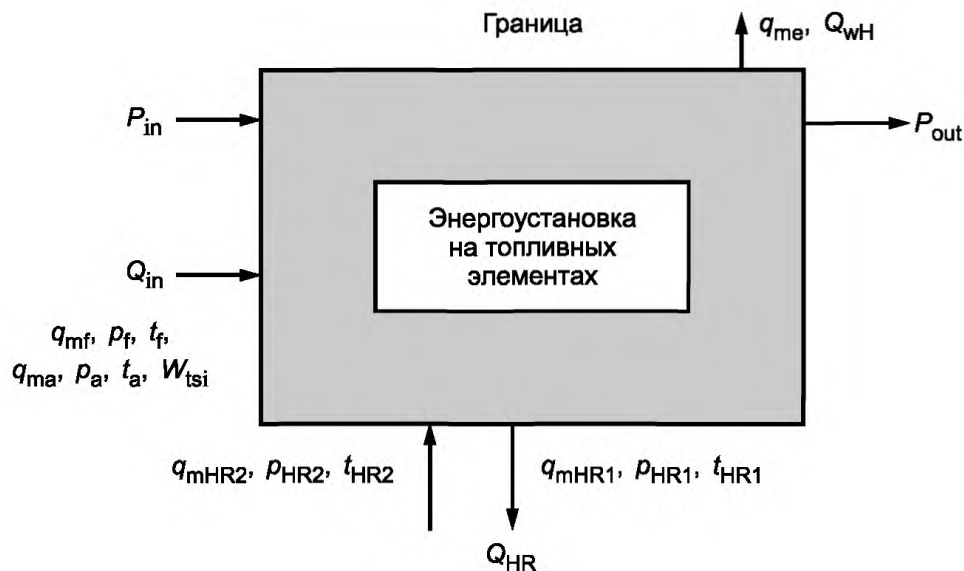
Рисунок 2 — Схема
