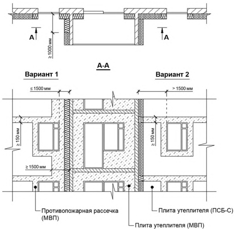
Рис. 9. Участки наружных стен по периметру остекленных лоджий (боковые торцы лоджий глухие)
