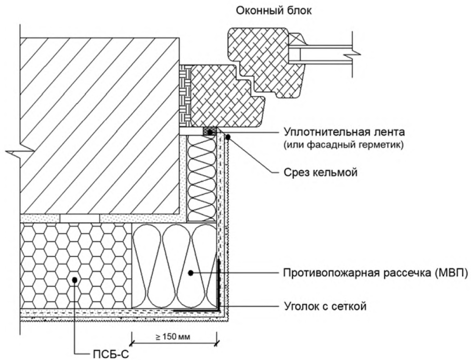
Рис. 6. Утеплитель и окантовки боковых откосов проемов
