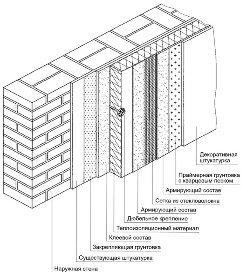
Рис. 1. Основные составляющие СФТК
