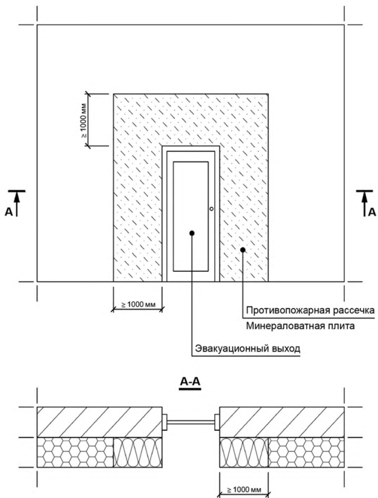
Рис. 7. Участки наружных стен по периметру эвакуационных выходов из здания
