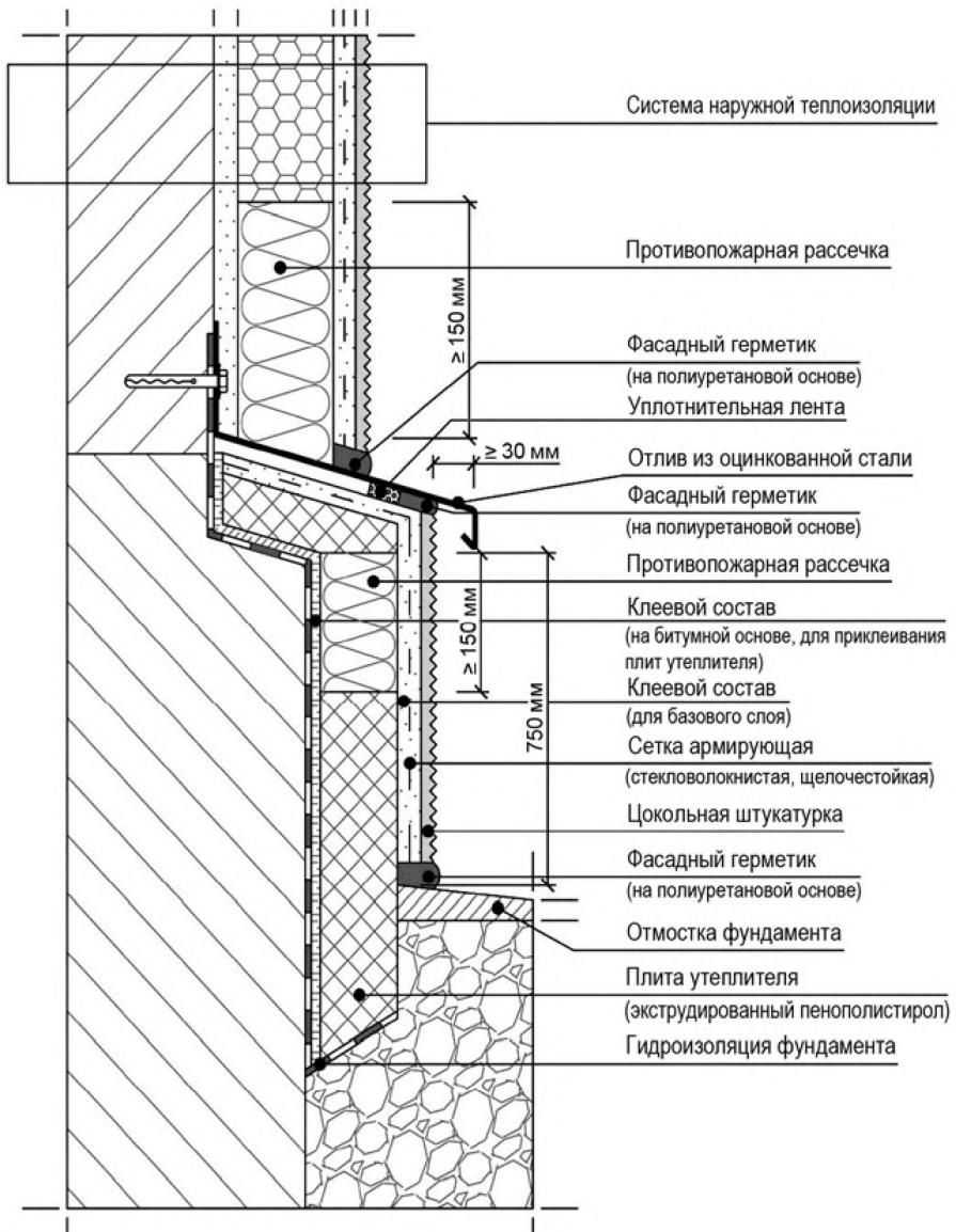
Рис. 19. Участки примыкания СФТК к цоколю здания
