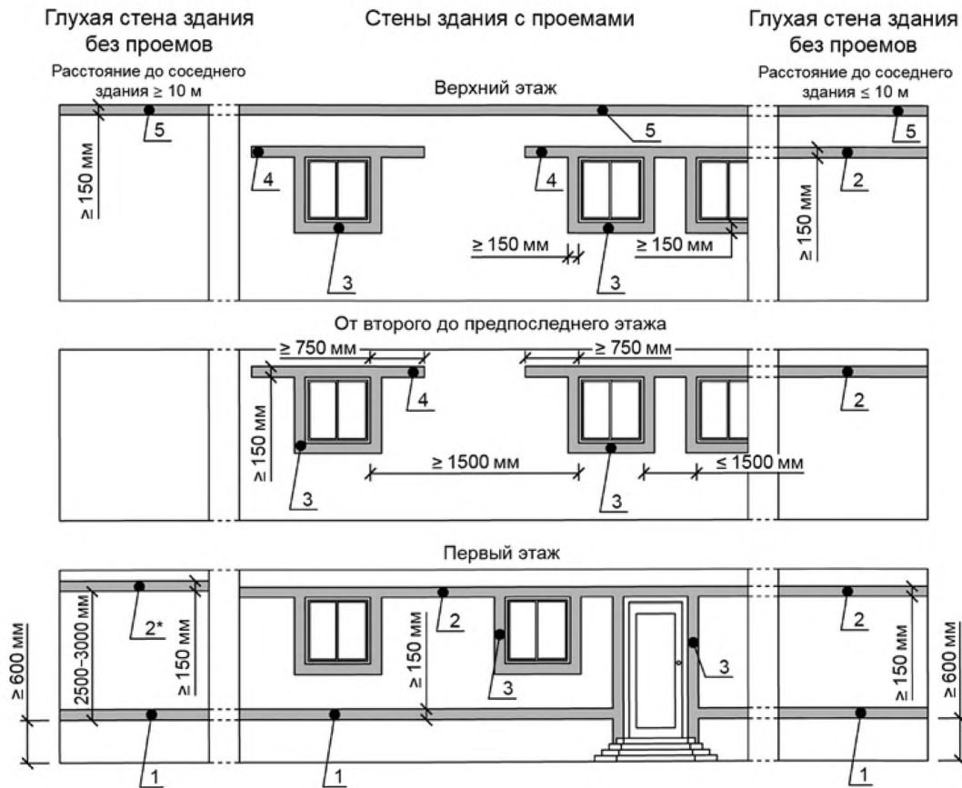
Рис. 13. Участки наружных стен здания с поэтажными рассечками и обрамлением проемов из МВЛ
