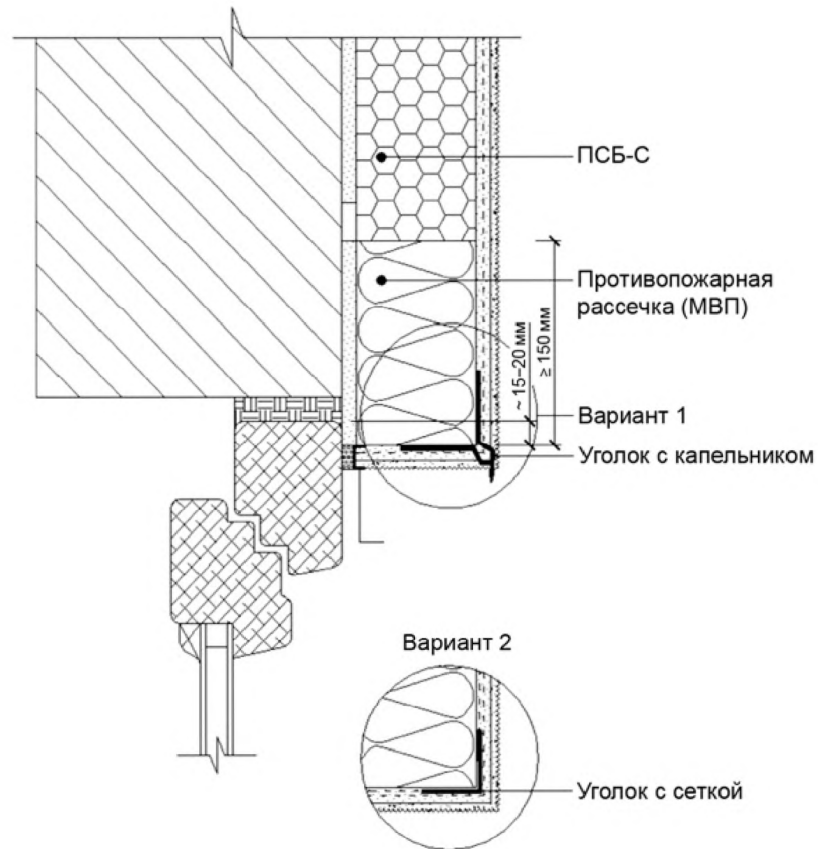
Рис. 5. Утеплитель и окантовки верхних откосов проемов
