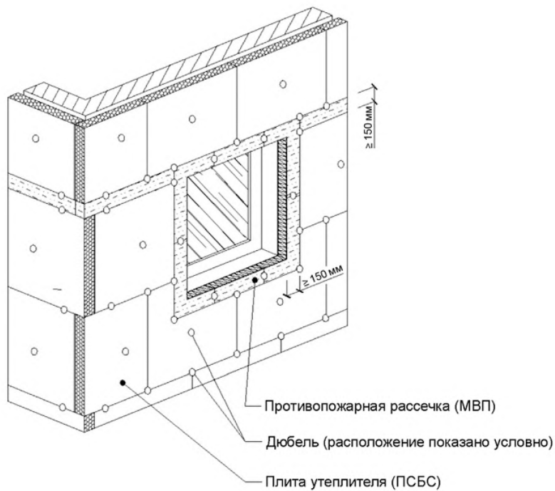
Рис. 4. Утеплитель, противопожарные рассечки и окантовки проемов
