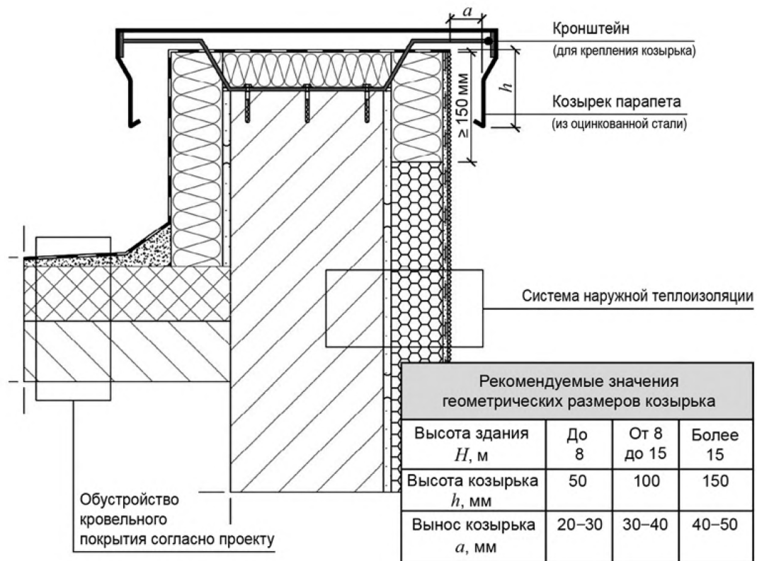
Рис. 16. Участки примыкания СФТК к парапету здания
