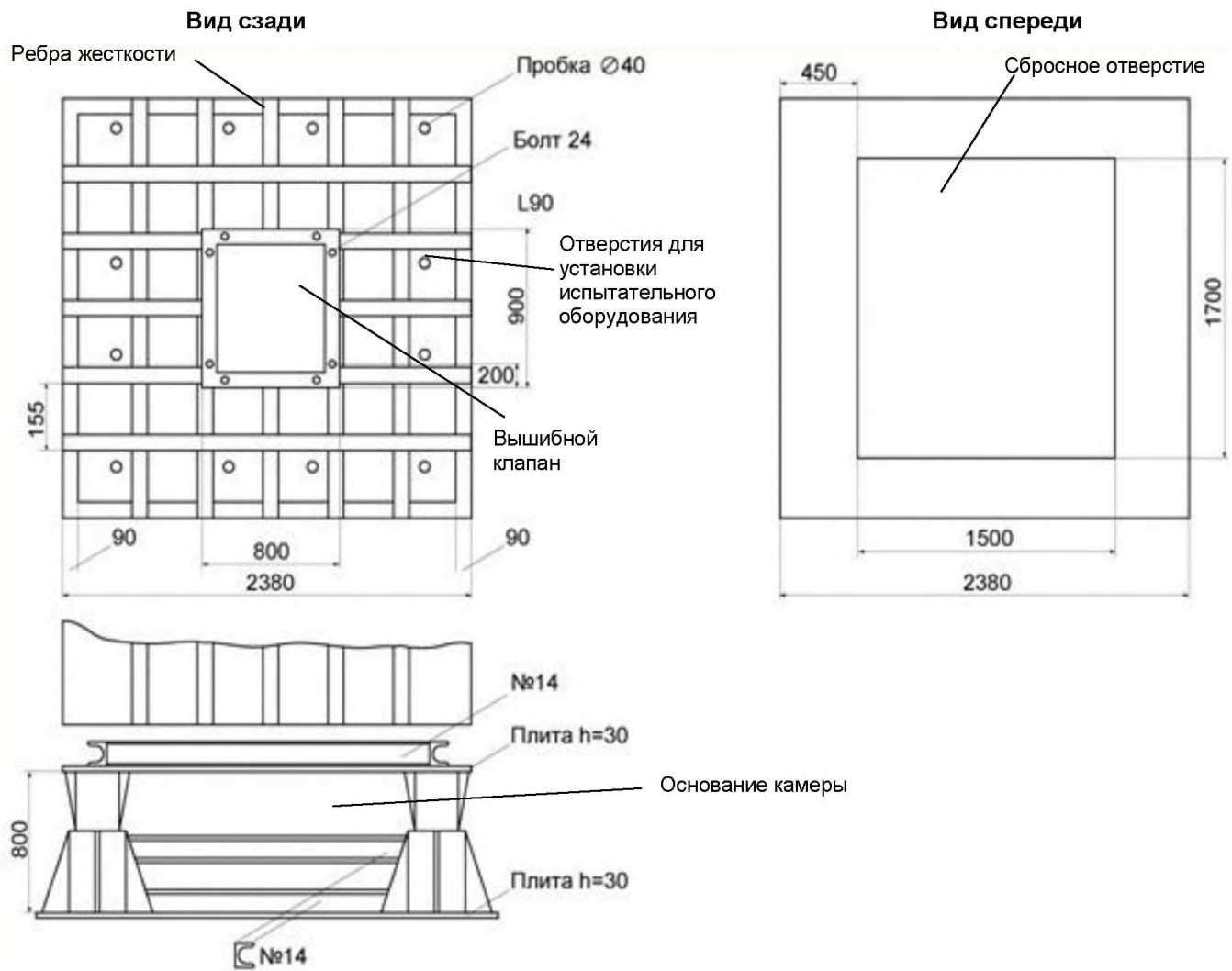
Рисунок А.1 – Схема испытательной взрывной камеры
