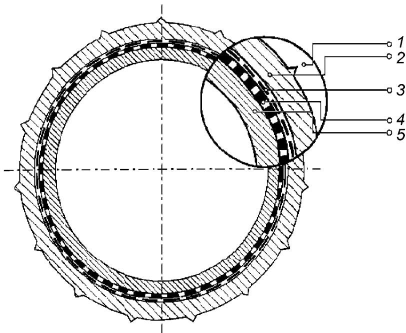
1 — горная порода; 2 — торкрет-бетон; 3 — геотекстиль; 4 — геосинтетический гидроизоляционный материал; 5 — бетон
