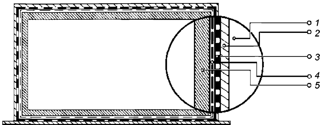
1 — горная порода; 2 — защитный слой; 3 — геотекстиль; 4 — геосинтетический гидроизоляционный материал; 5 — бетон
