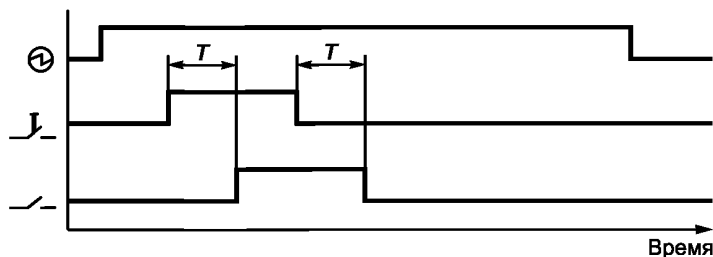
⊕ — источник электропитания; J — сигнал управления; T — установленное время; \text{—/—} — главный контакт
