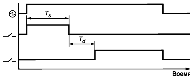
⊙ — источник электропитания; T_s — время установки звезды; T_d — время треугольника; — — главный контакт
