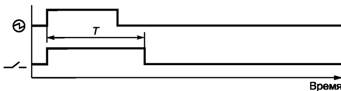
Рисунок 14 — Реле времени на удержание
