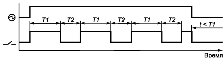
⊙ — источник электропитания; T_1 — время импульса; T_2 — время паузы; — — главный контакт
