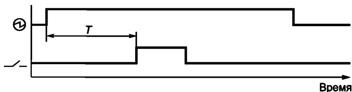
Рисунок 8 — Импульсное реле с задержкой
