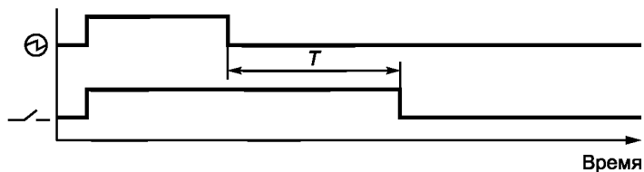
⊕ — источник электропитания; T — установленное время; \text{—/—} — главный контакт
