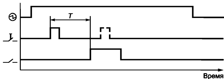
Рисунок 9 — Импульсное реле с задержкой по управляющему сигналу
