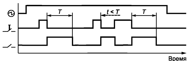
Рисунок 13 — Перезапускаемое интервальное реле с включением по управляющему сигналу
