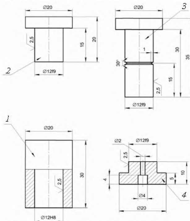
Рисунок 7– Металлическая форма для изготовления сырцовых гранул
