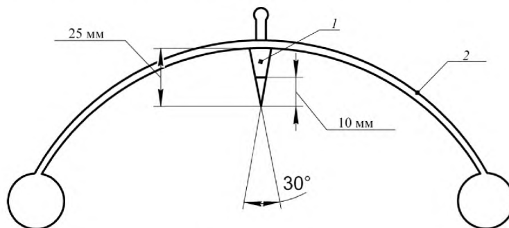
1 – балансирный конус; 2 – коромысло с балансируемыми шариками
