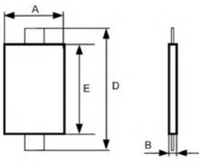
ф – плоский аккумулятор (2)
