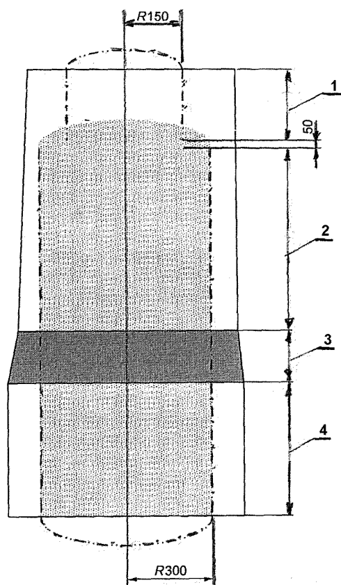
Рисунок 101 — Точки измерений для приборов, которые устанавливаются над человеком
