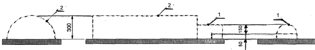
Рисунок 101 — Точки измерений для приборов, которые устанавливаются над человеком
