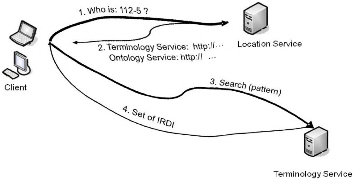
Рисунок 4 — Пример поиска концепций на Уровне 2
