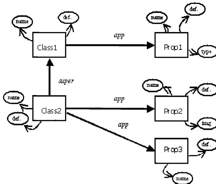
Рисунок Е.4—Результаты запрашивания объекта get_concept_model , пример 3
