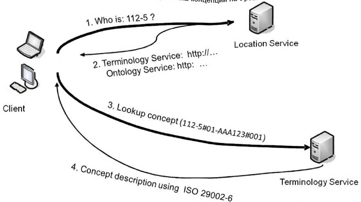
Рисунок 5 — Пример поиска концепций по идентификатору на Уровне 2
