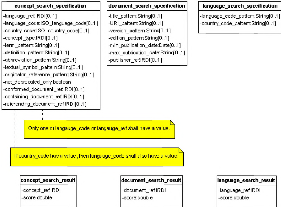
Рисунок 9 — Диаграмма класса UML для терминологической службы
