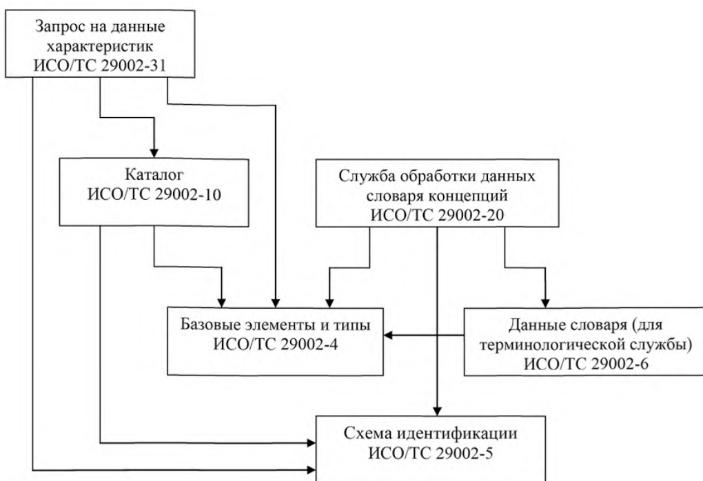
Рисунок 2 — Диаграмма зависимости частей и уровней
